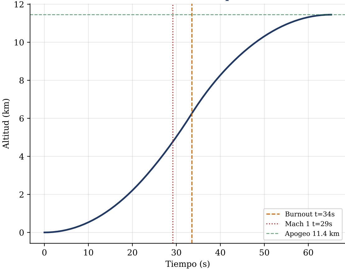
Altitud vs. Tiempo
