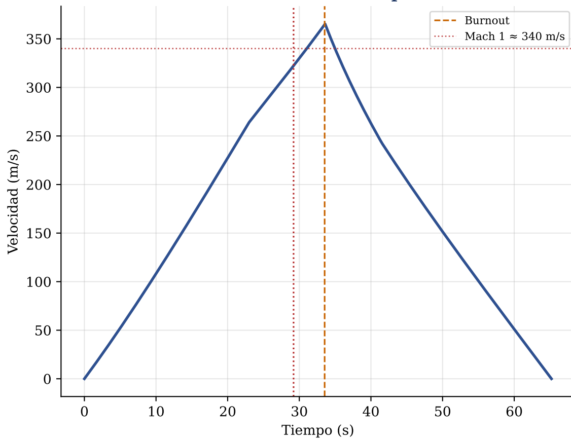
Velocidad vs. Tiempo
