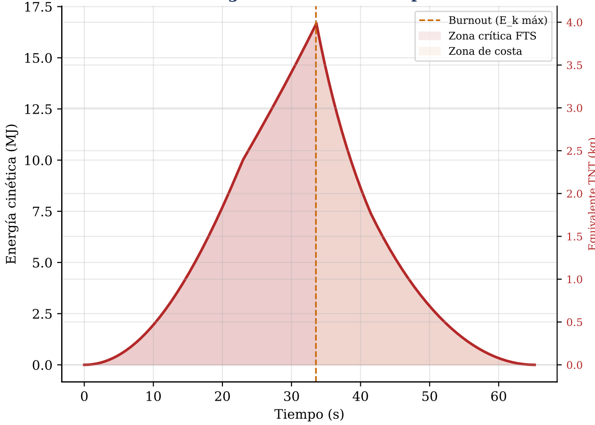
Energía Cinética vs. Tiempo
