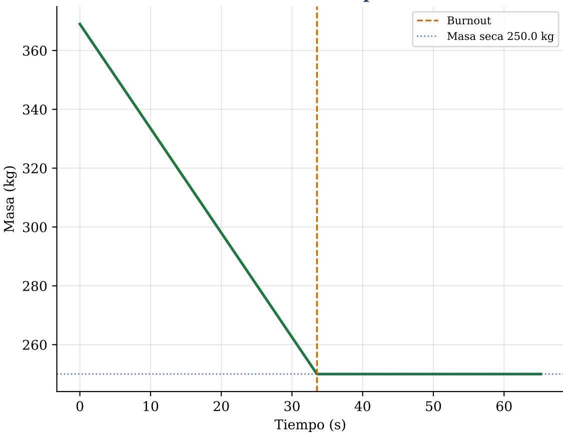
Masa vs. Tiempo
