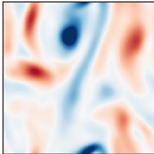
K = 200
