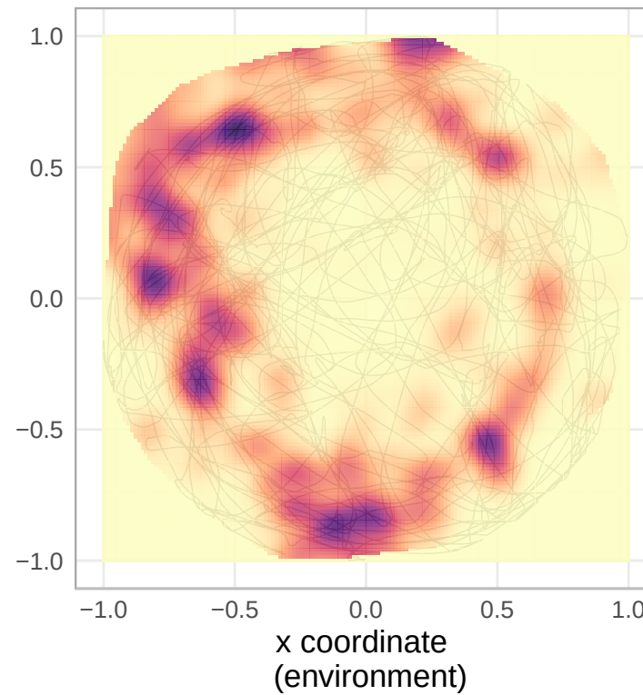
Neuron D
