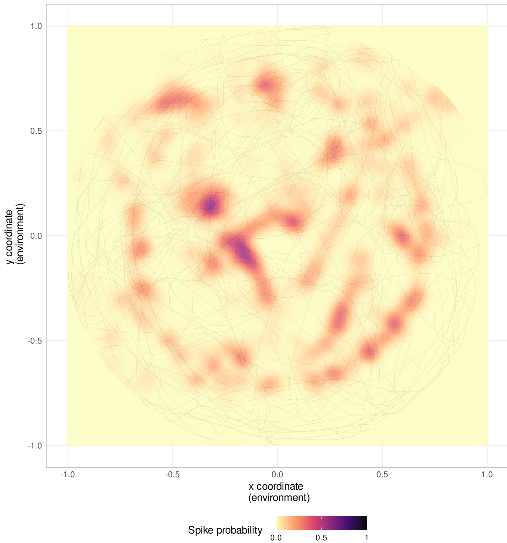
Neuron 124
