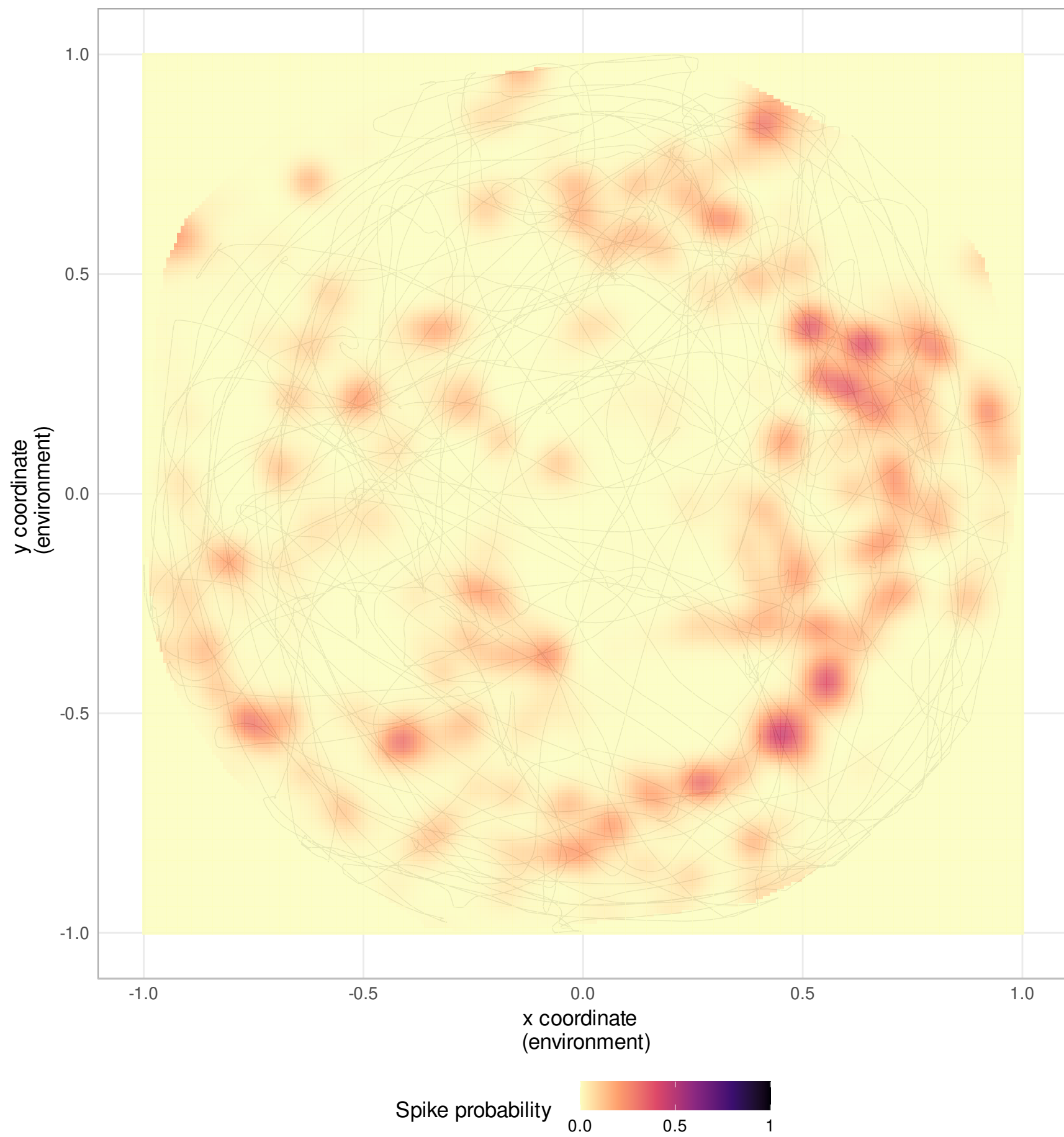
Neuron 134
