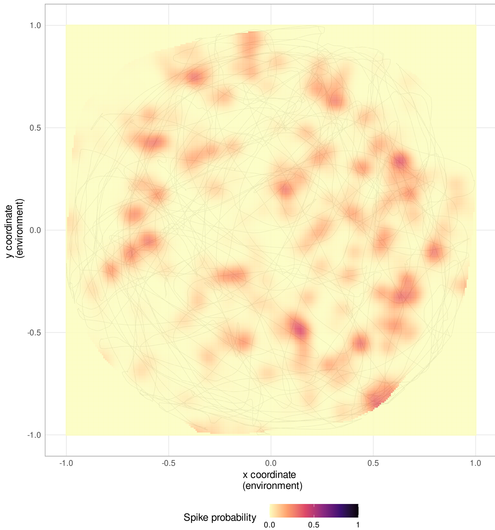
Neuron 137
