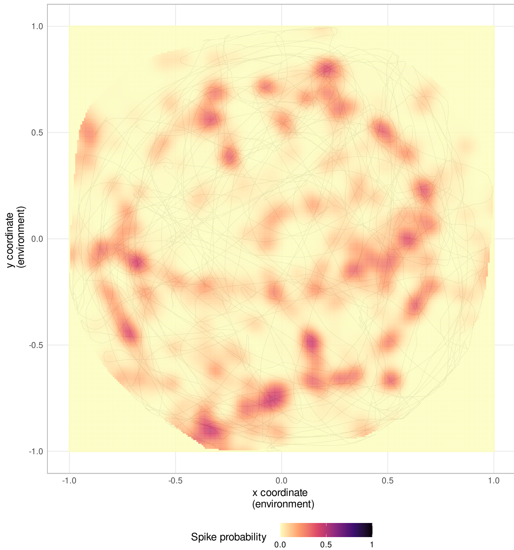
Neuron 145
