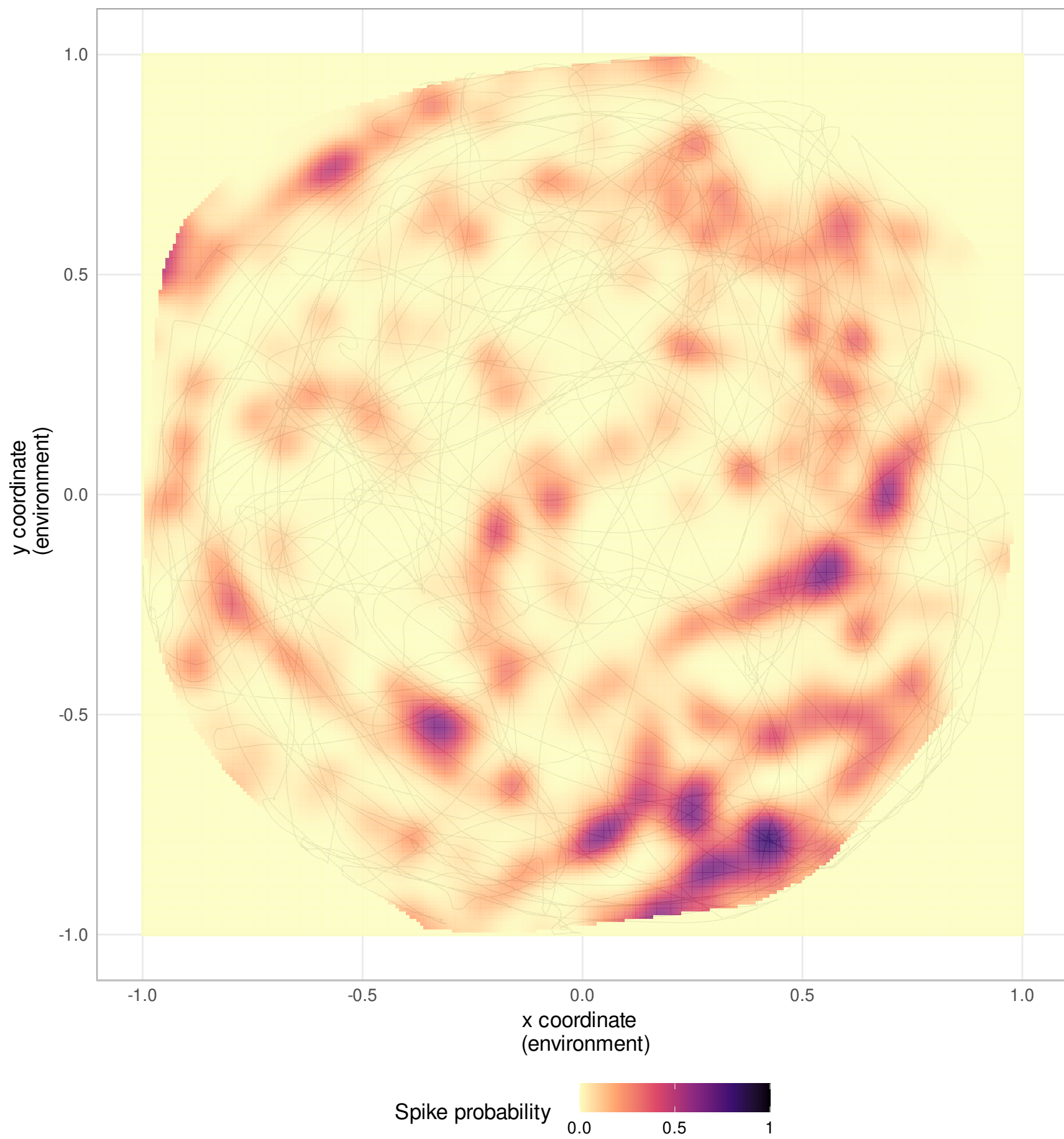
Neuron 15
