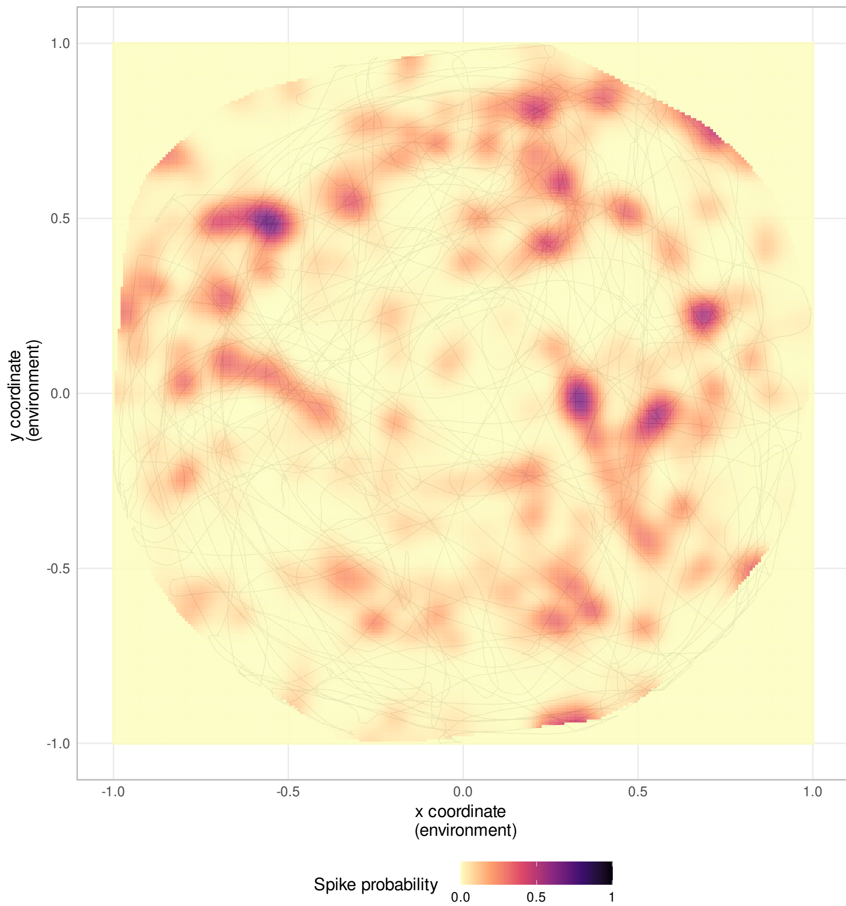
Neuron 156
