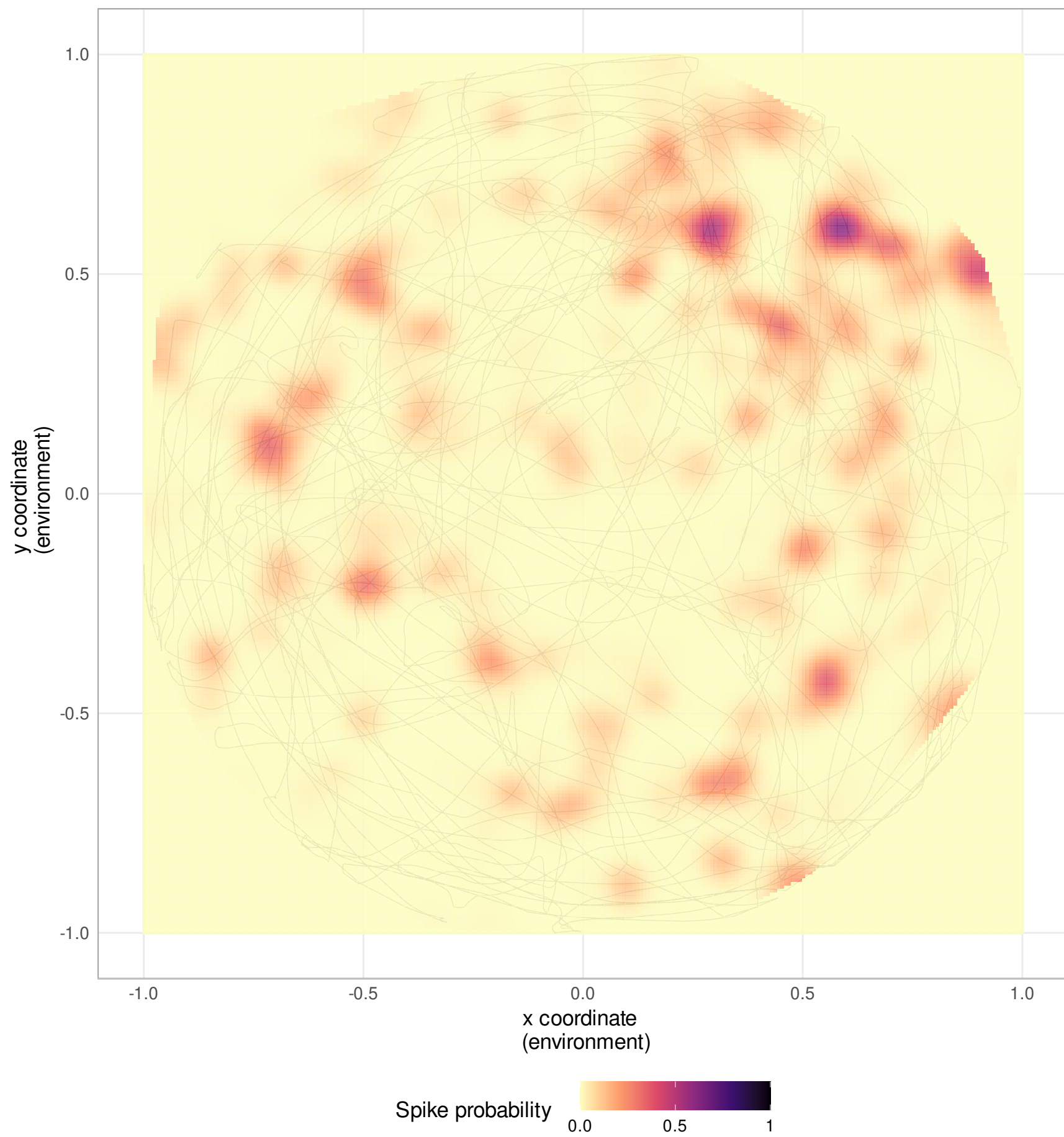
Neuron 157
