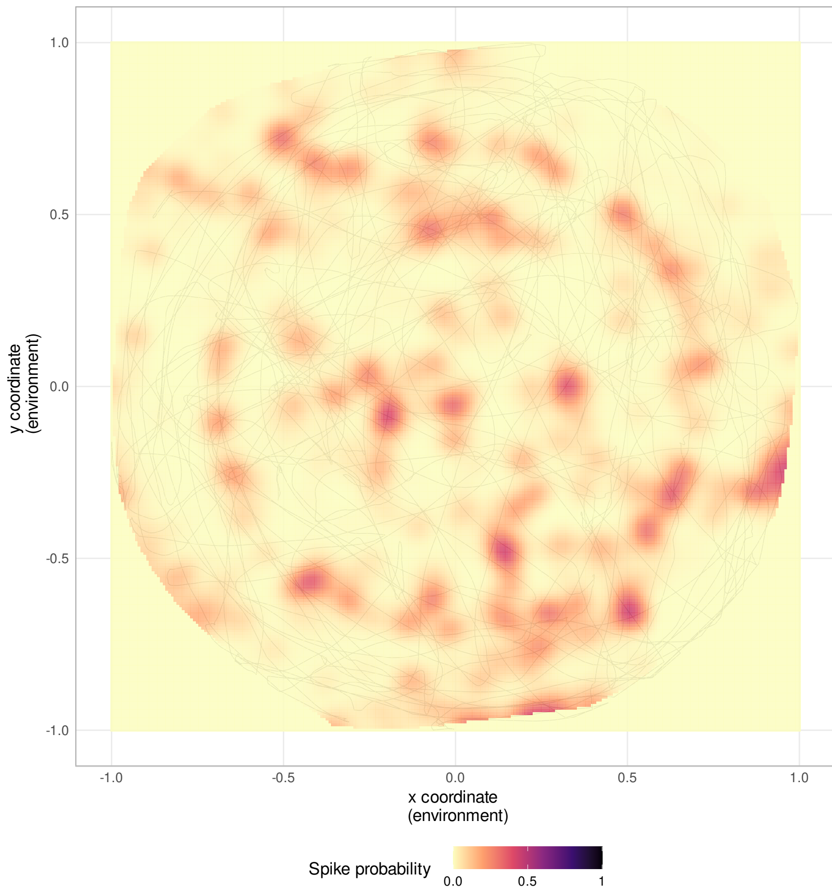
Neuron 161
