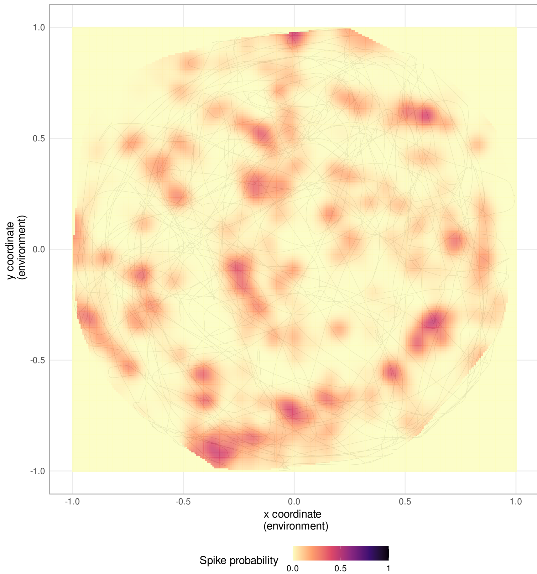
Neuron 171
