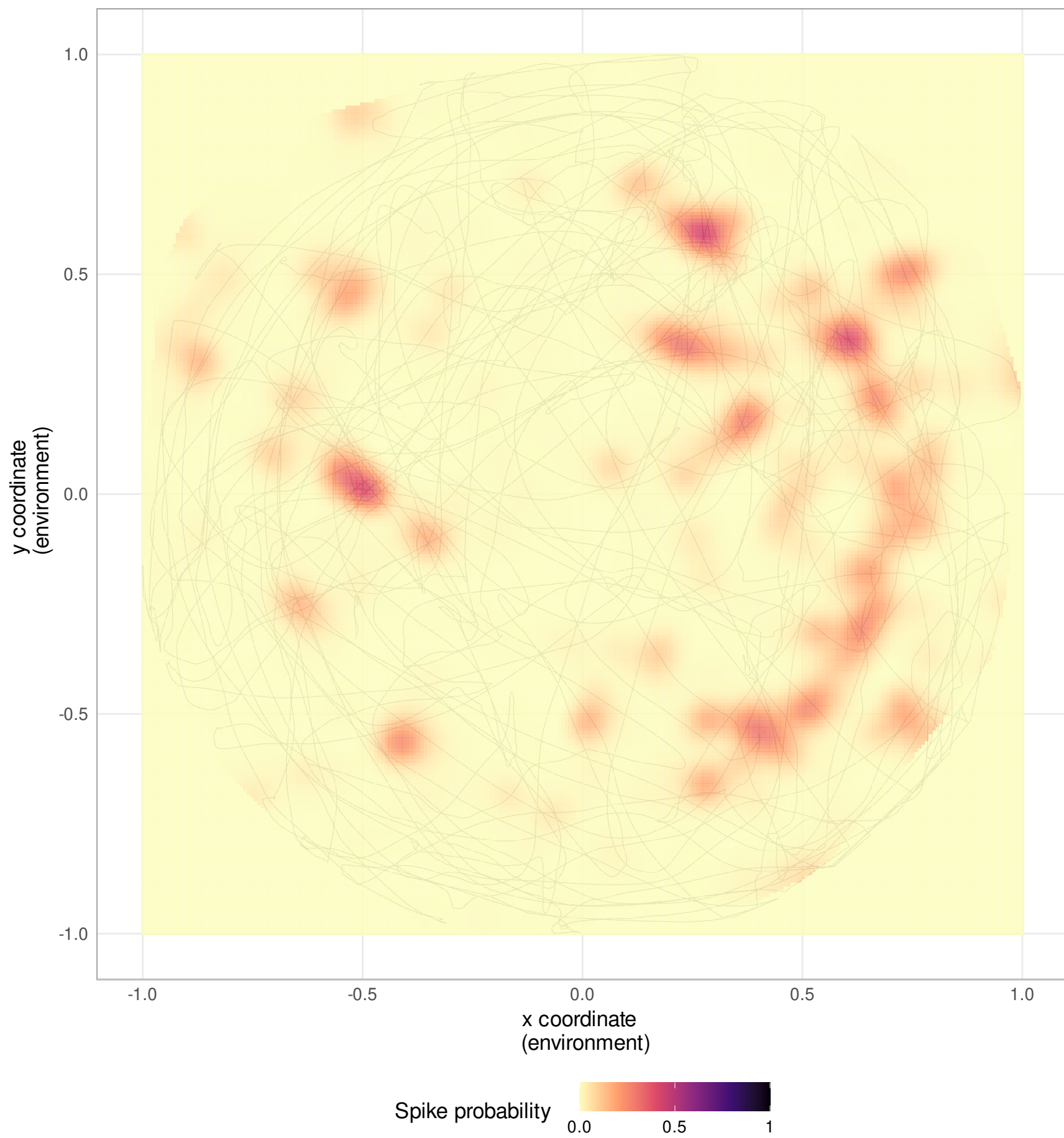
Neuron 174
