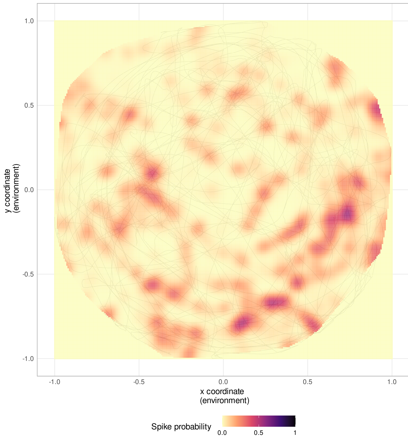
Neuron 183
