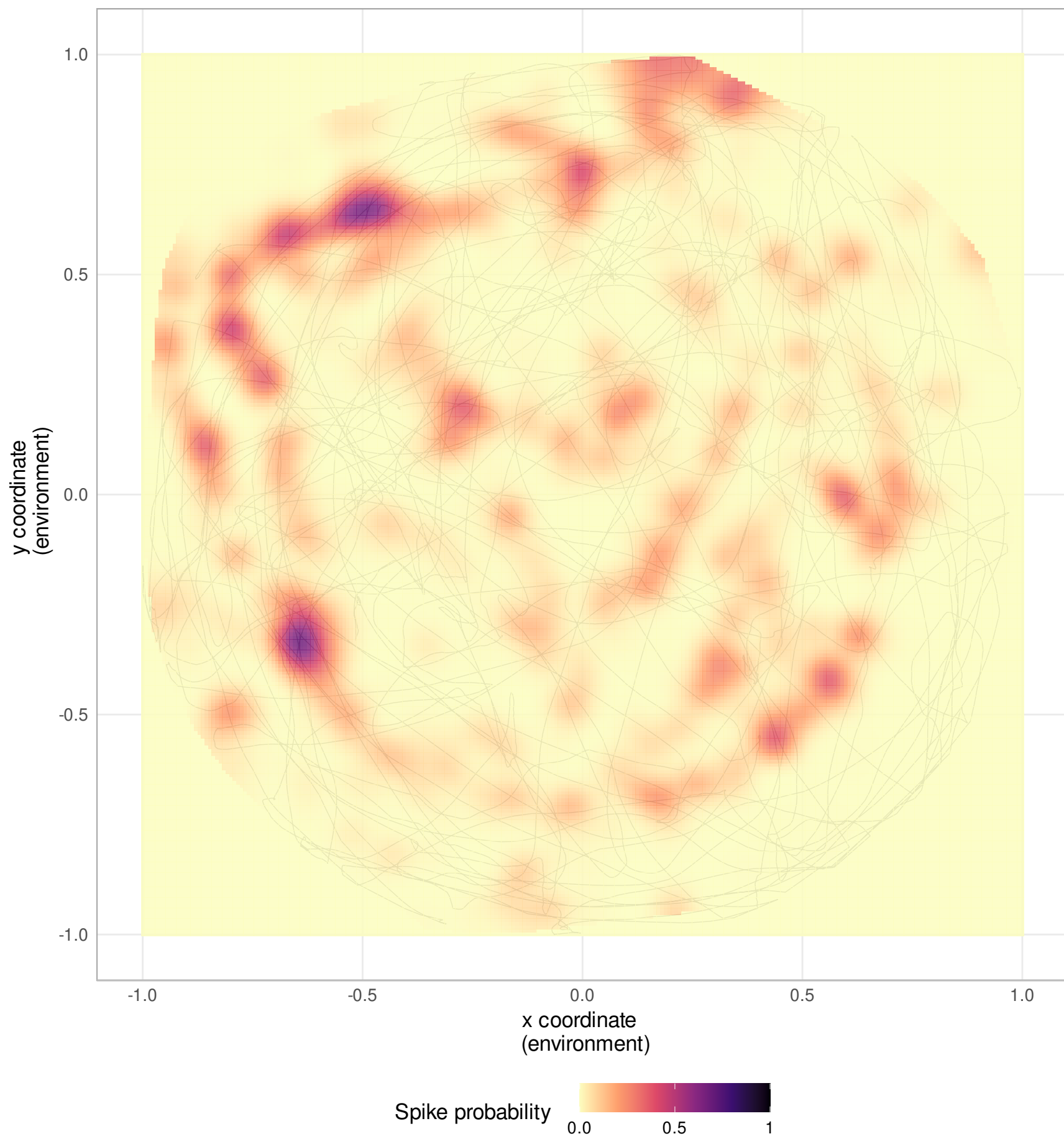
Neuron 203
