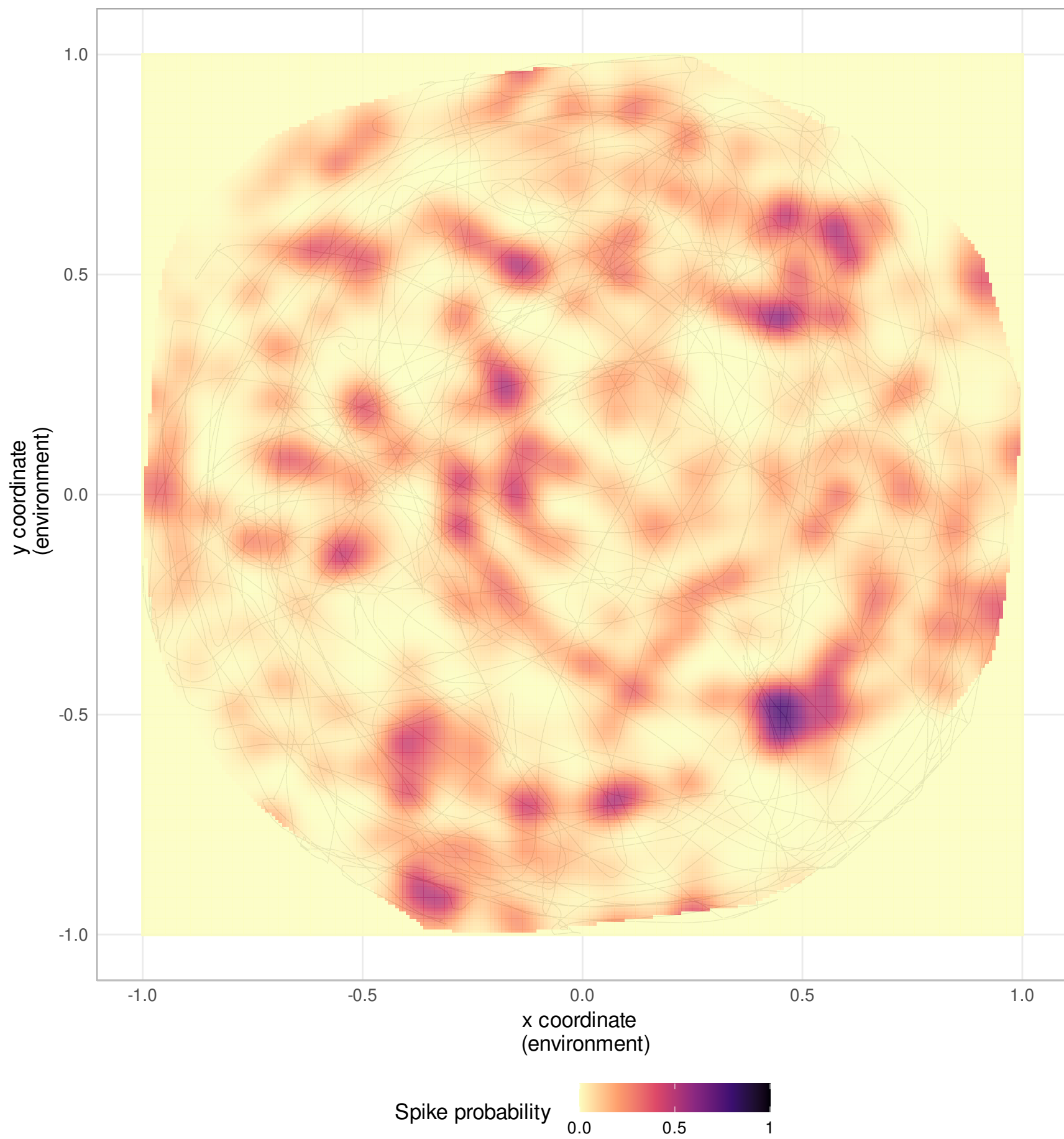
Neuron 206
