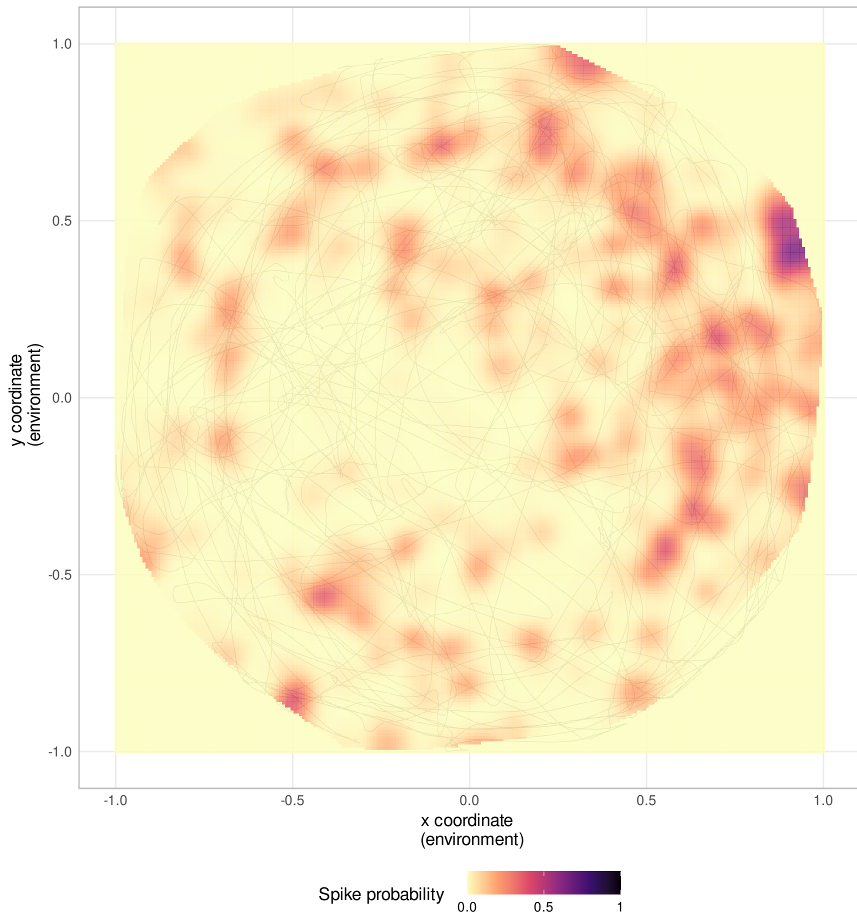
Neuron 209
