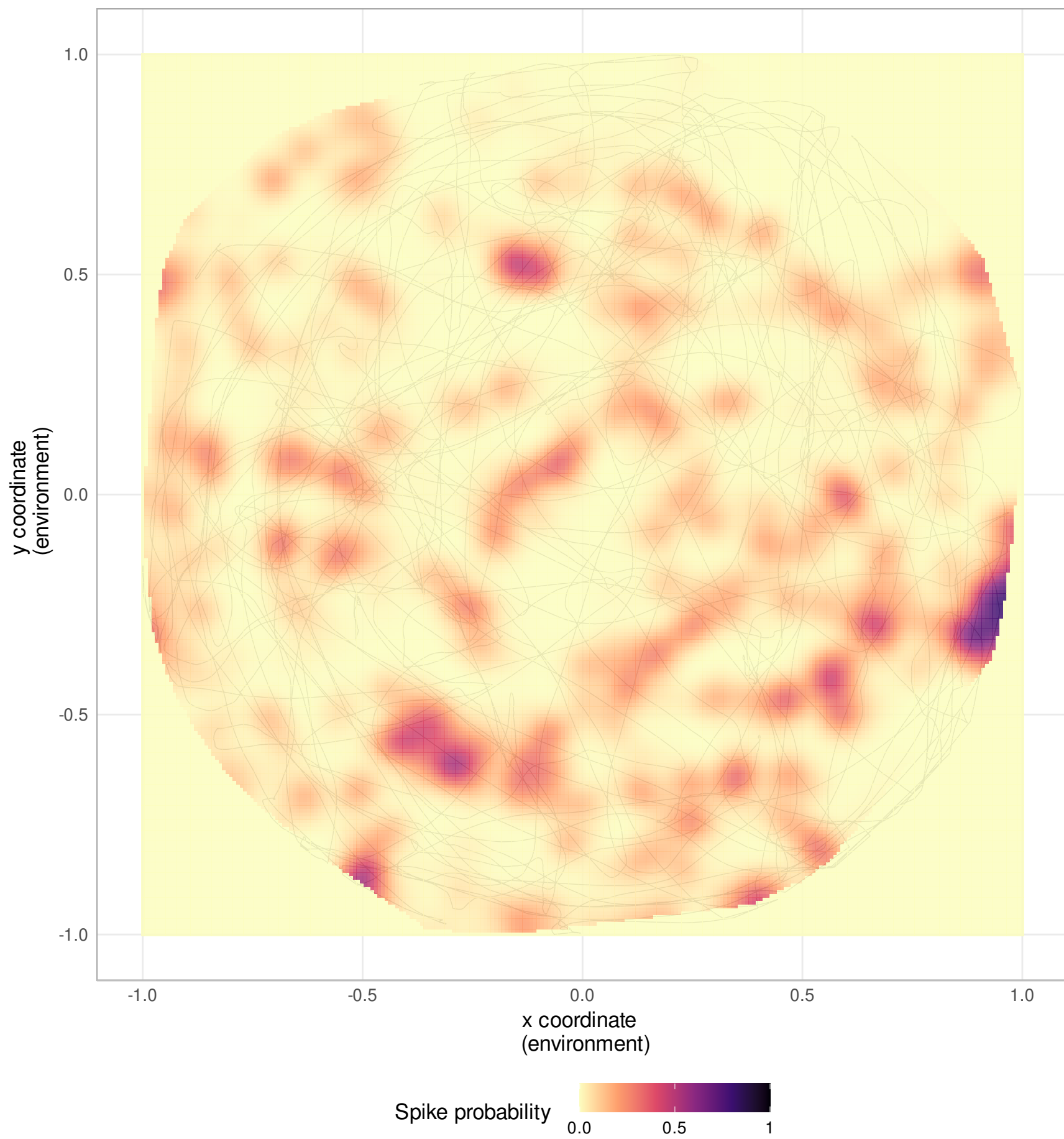
Neuron 220
