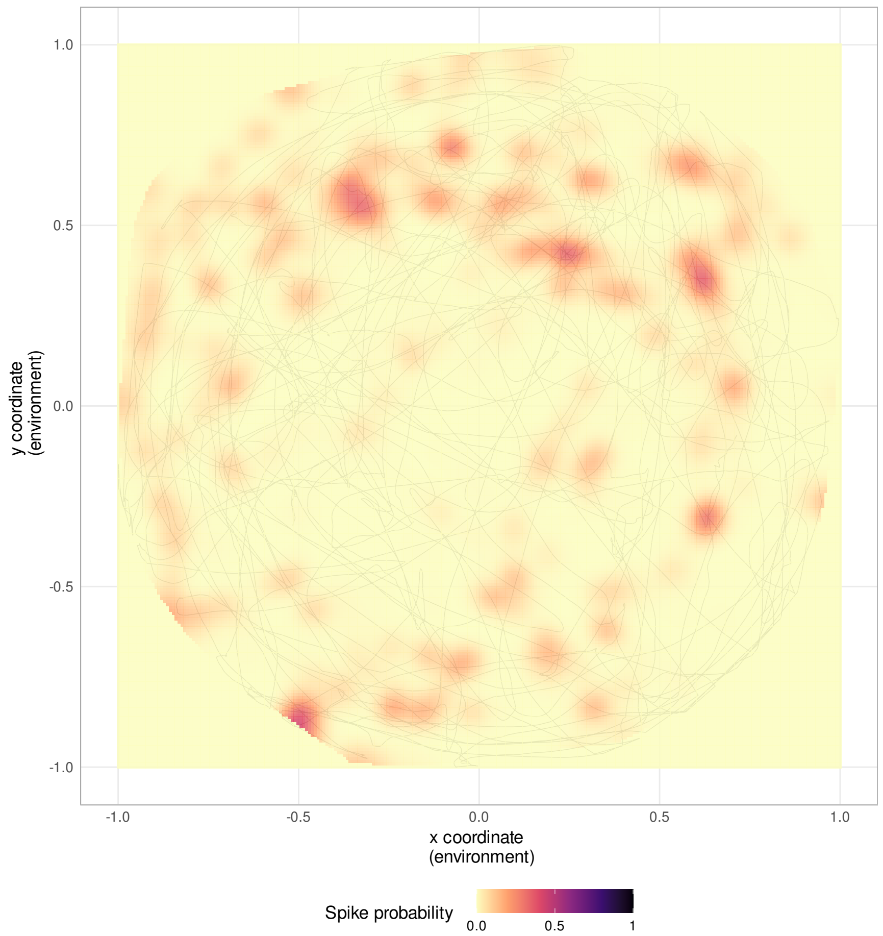
Neuron 223
