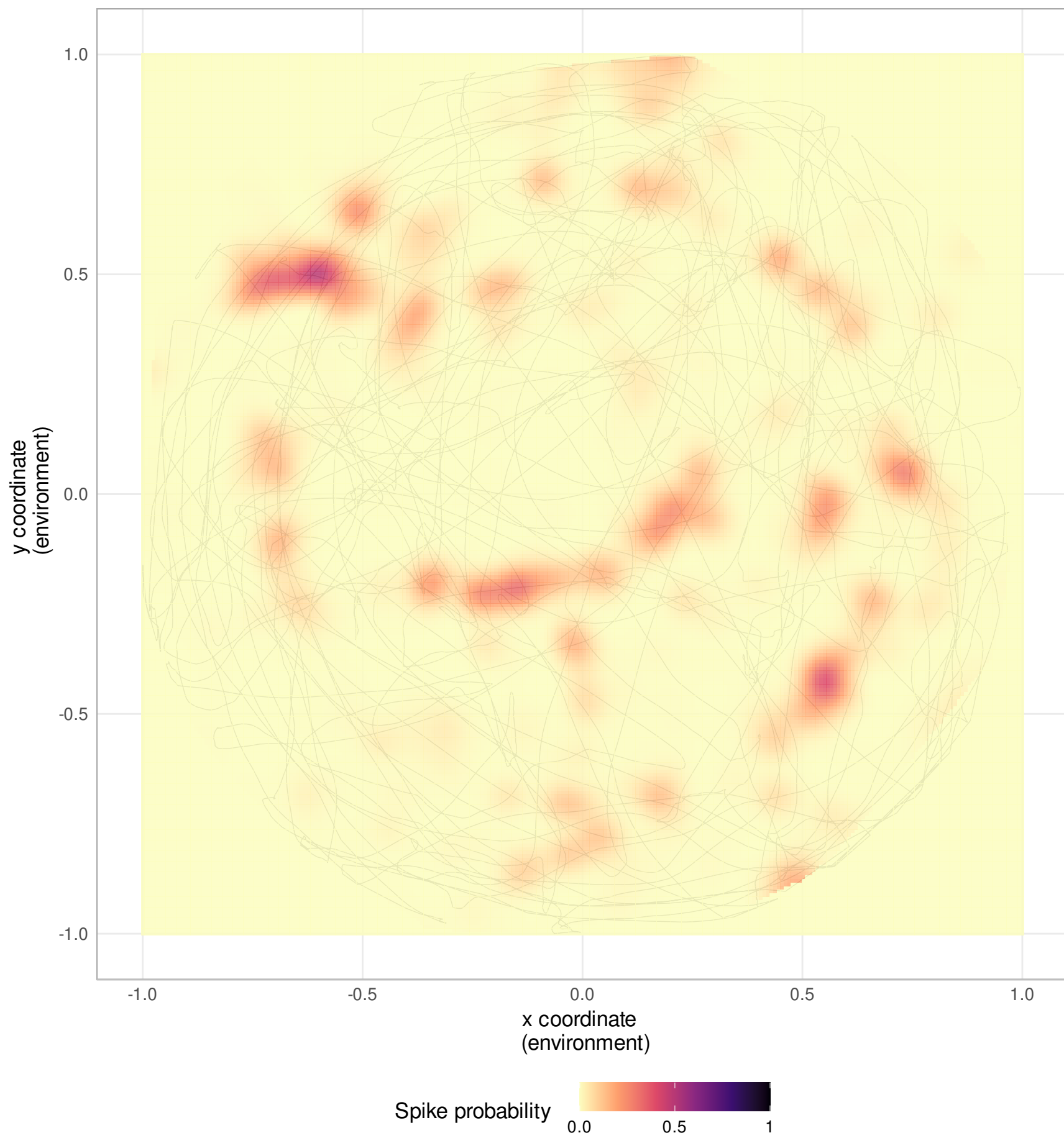
Neuron 224
