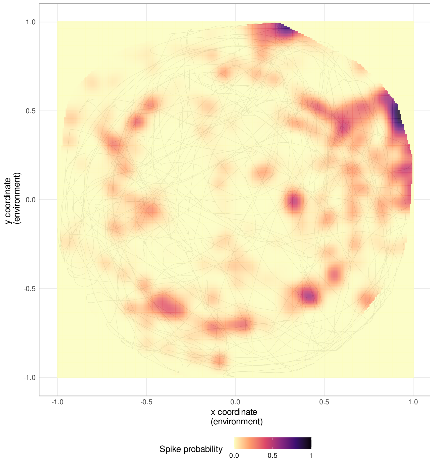
Neuron 229
