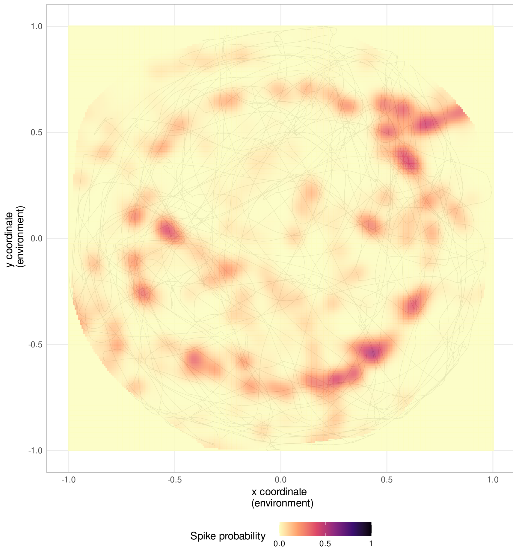
Neuron 237
