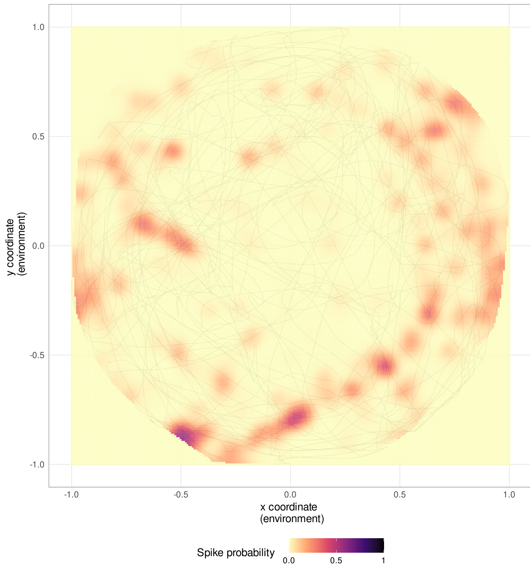
Neuron 242
