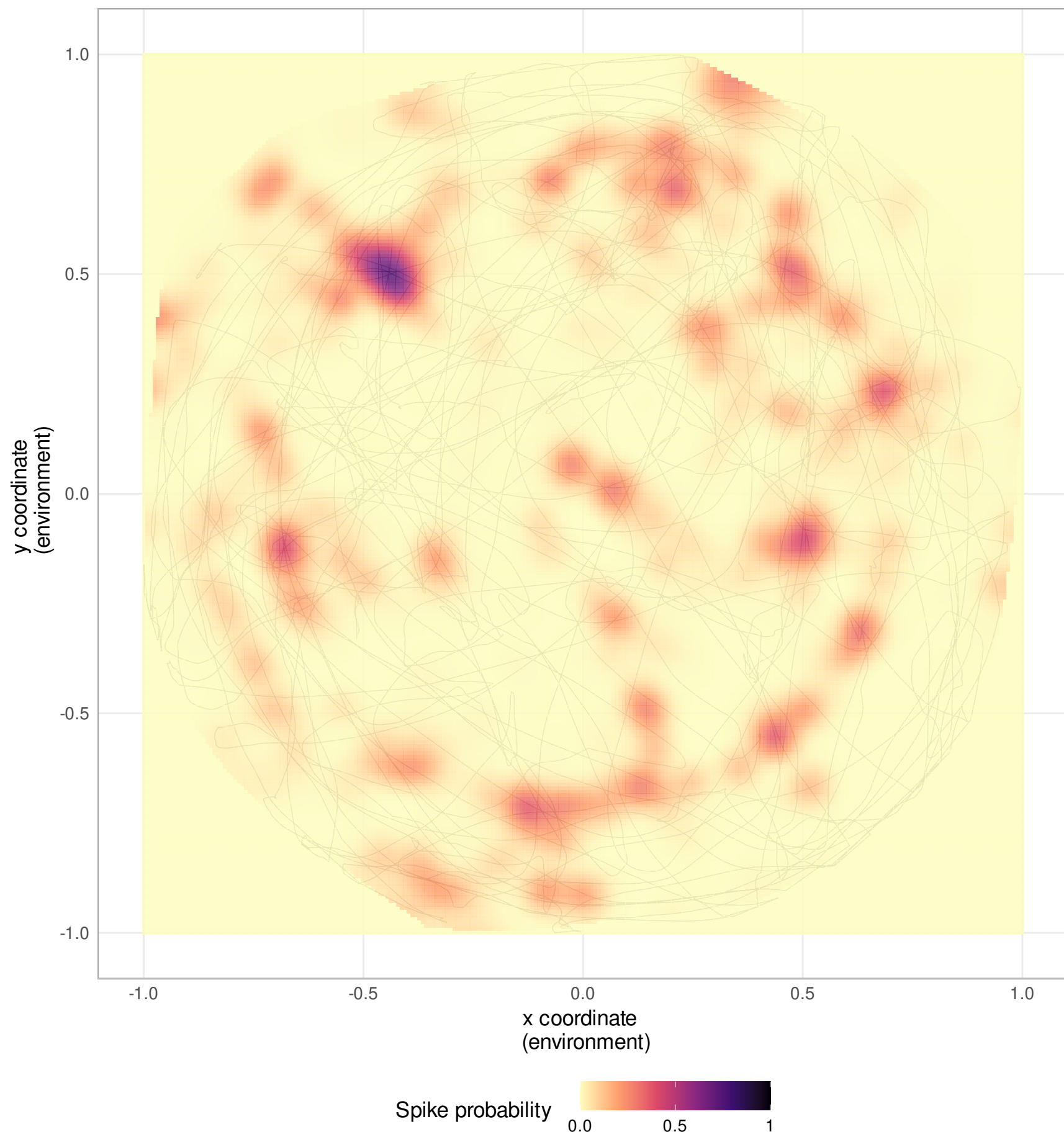
Neuron 243
