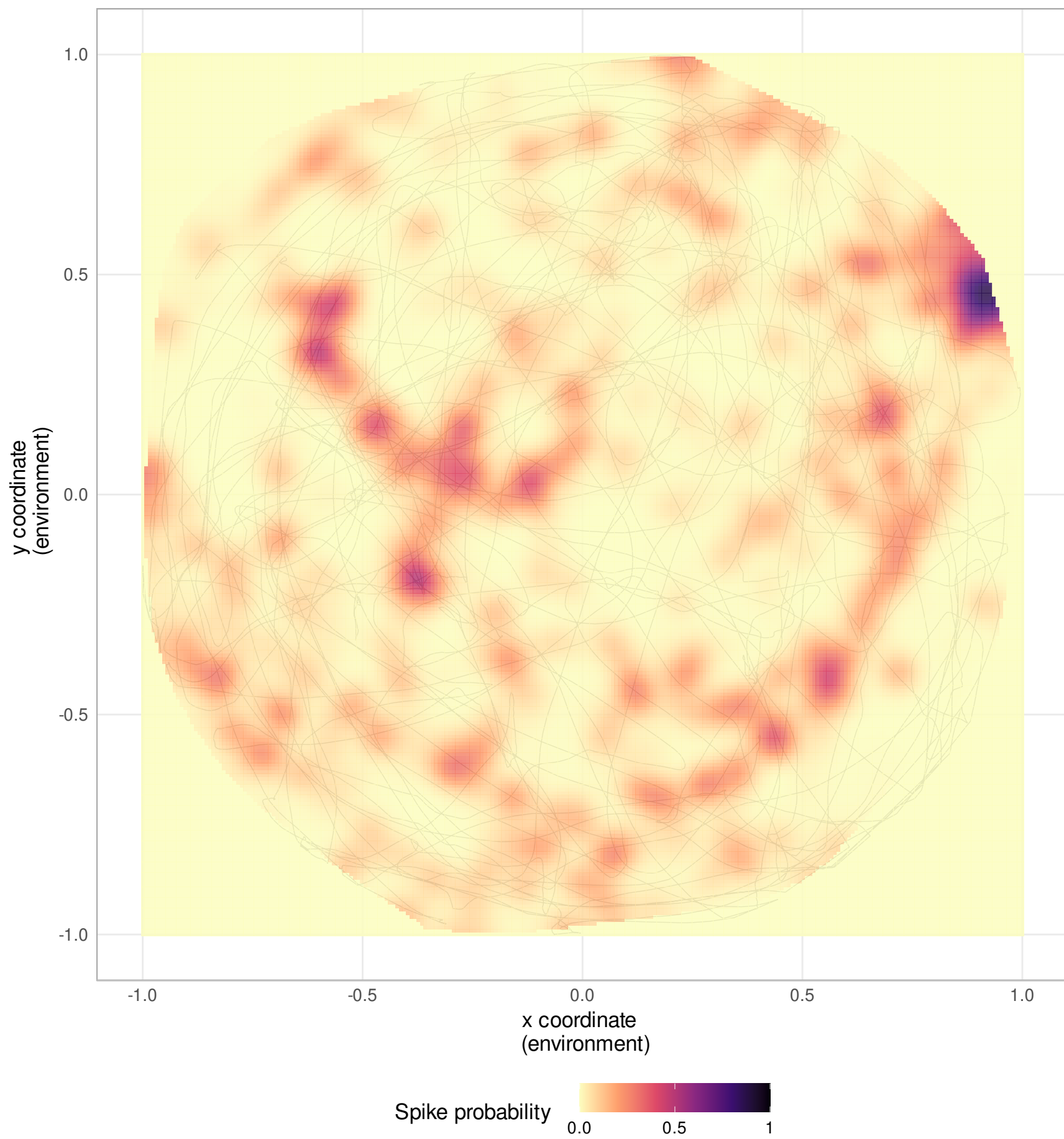
Neuron 246
