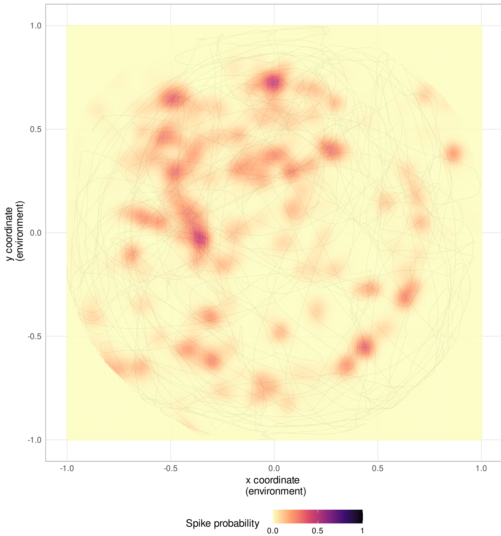
Neuron 248
