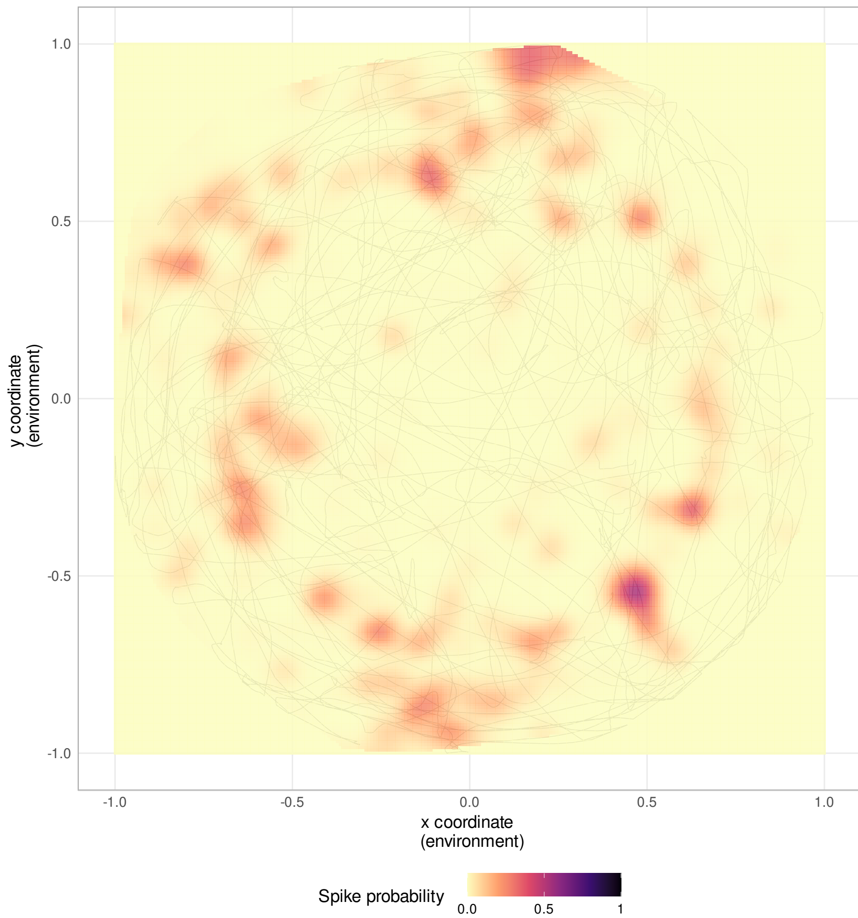
Neuron 255
