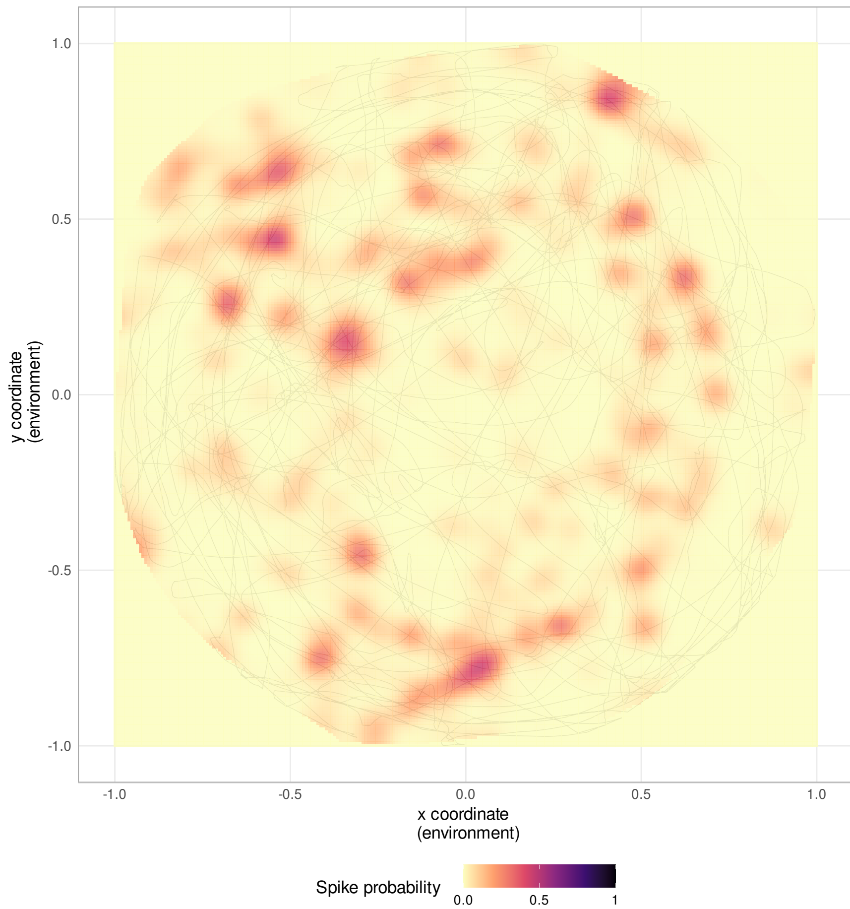
Neuron 269
