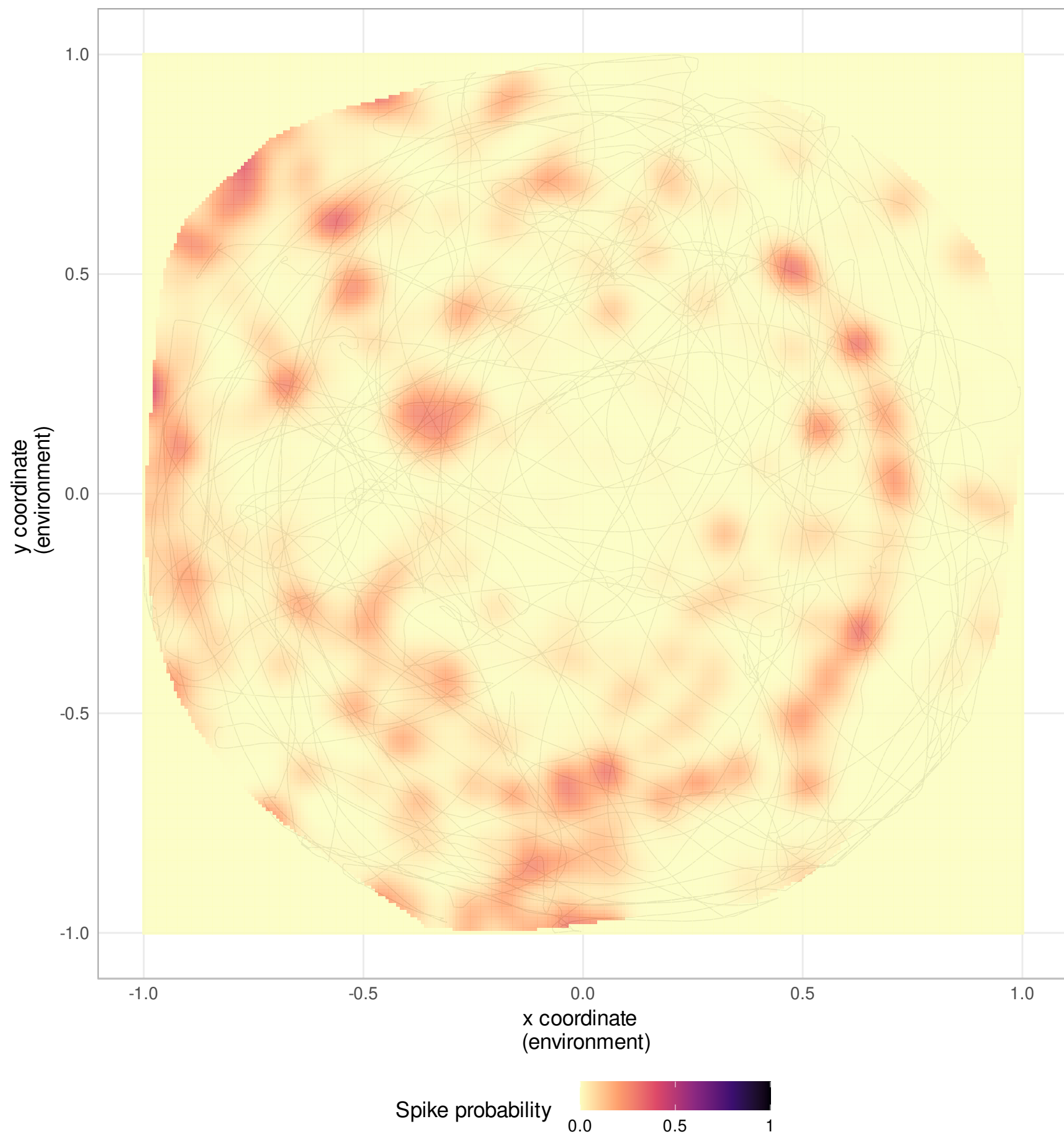
Neuron 273
