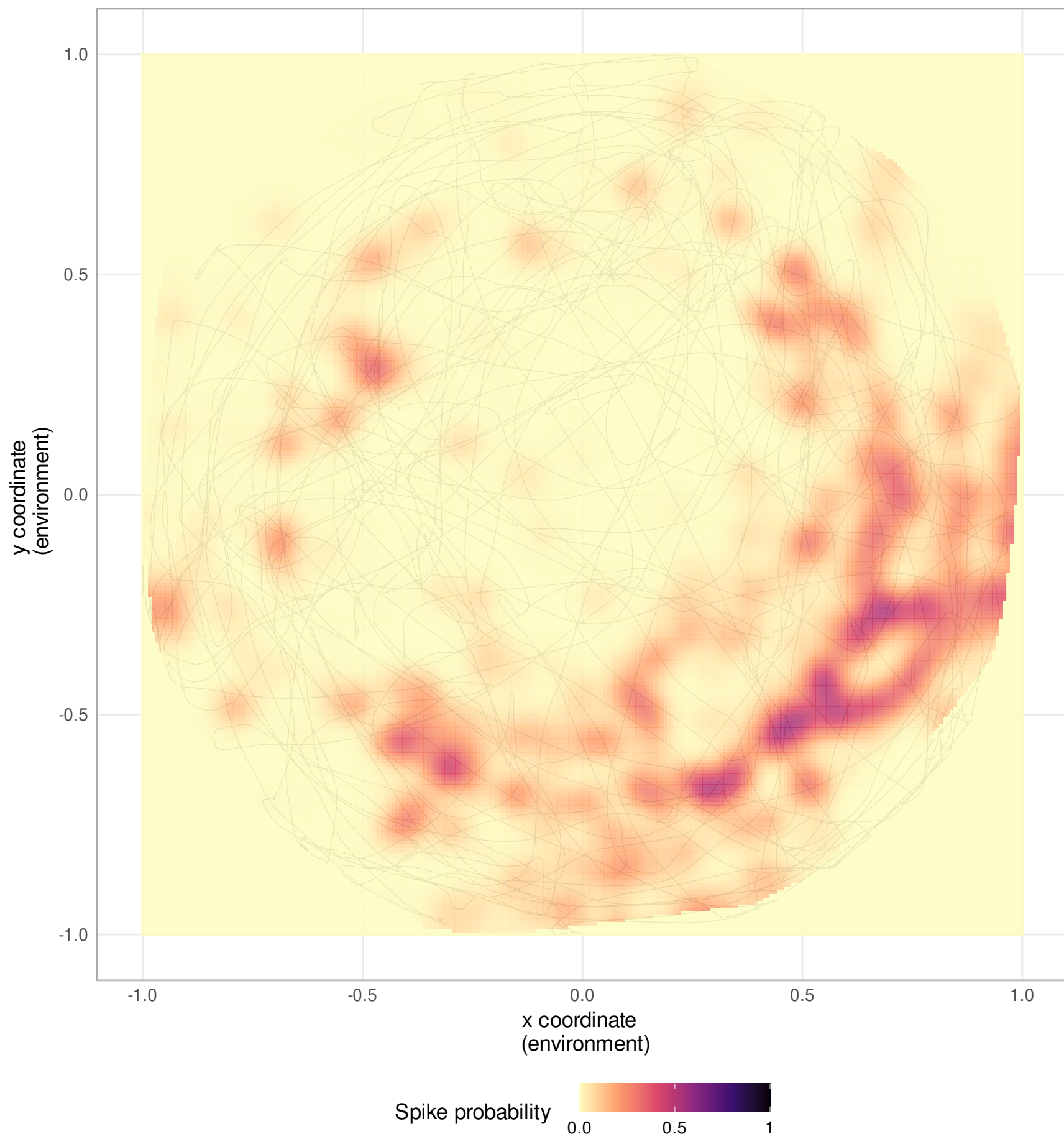
Neuron 277
