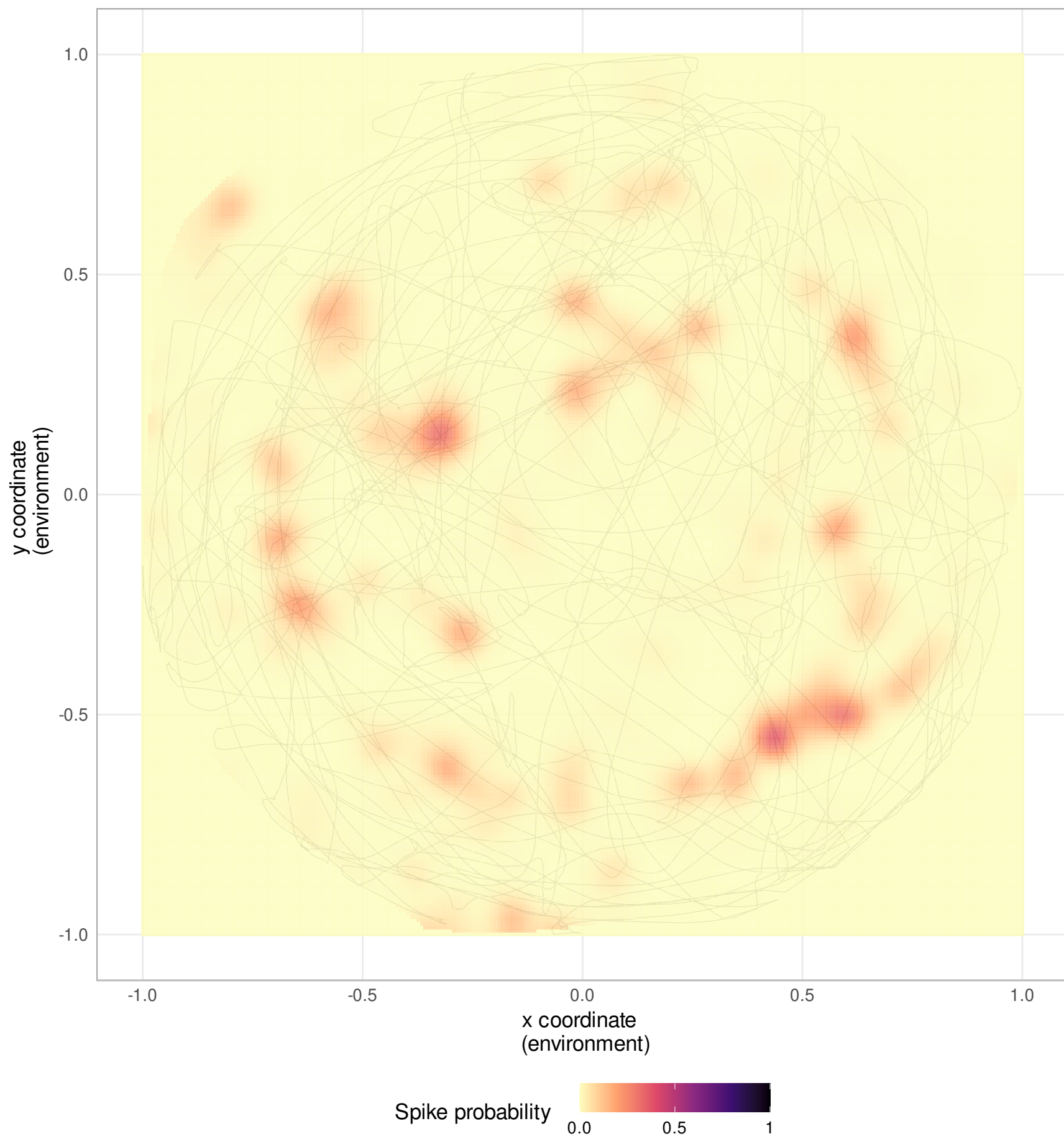
Neuron 281
