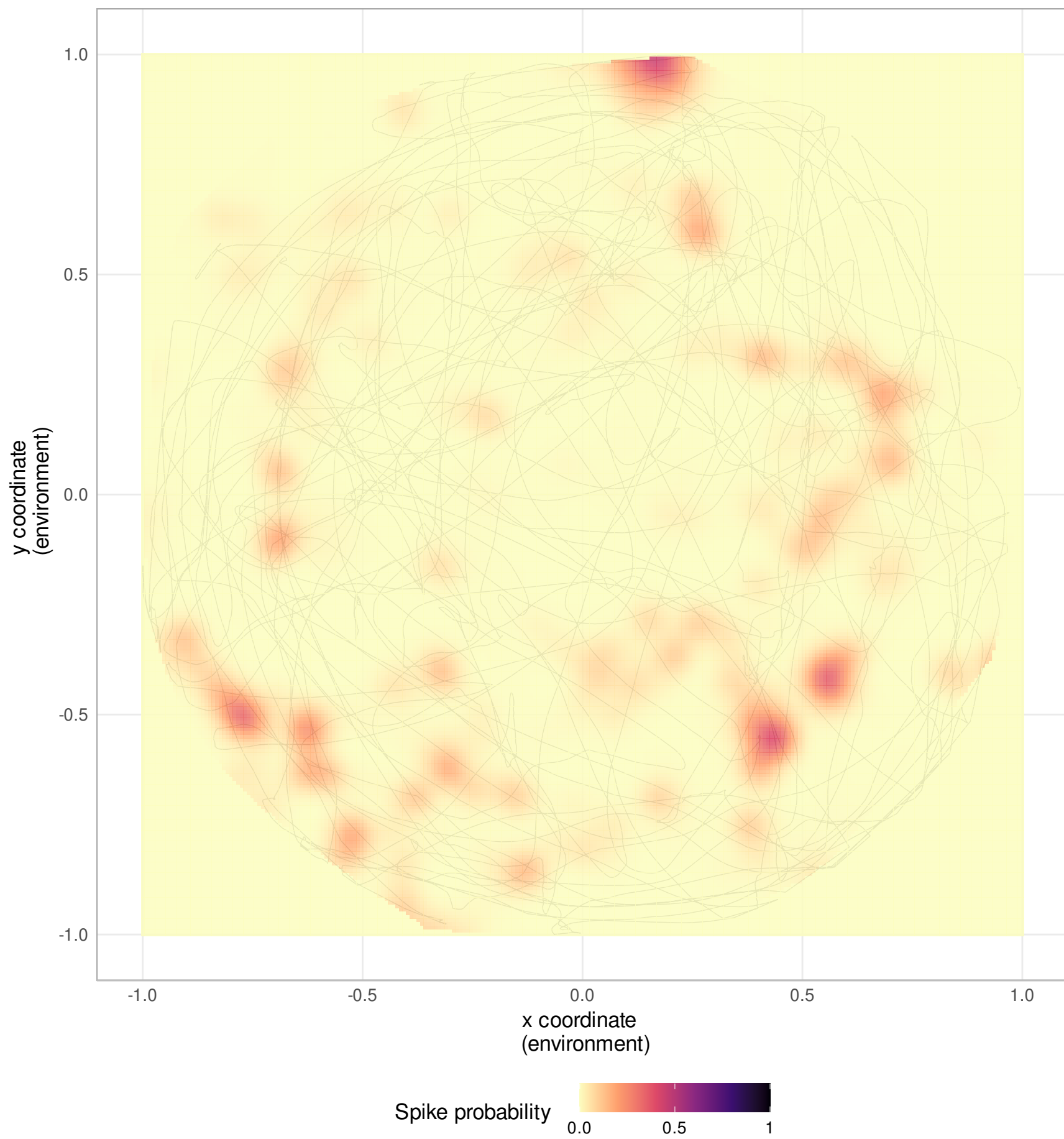
Neuron 282
