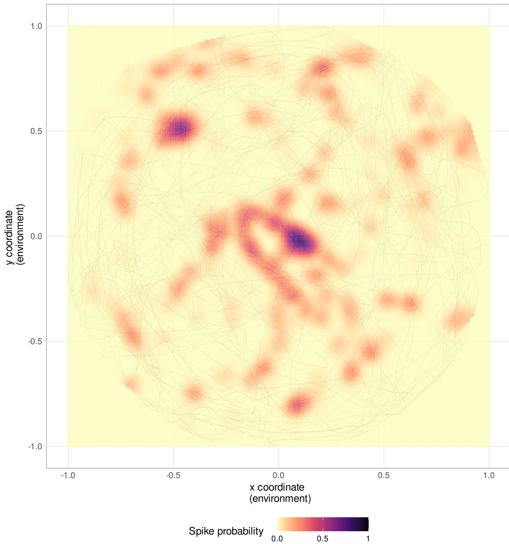
Neuron 285
