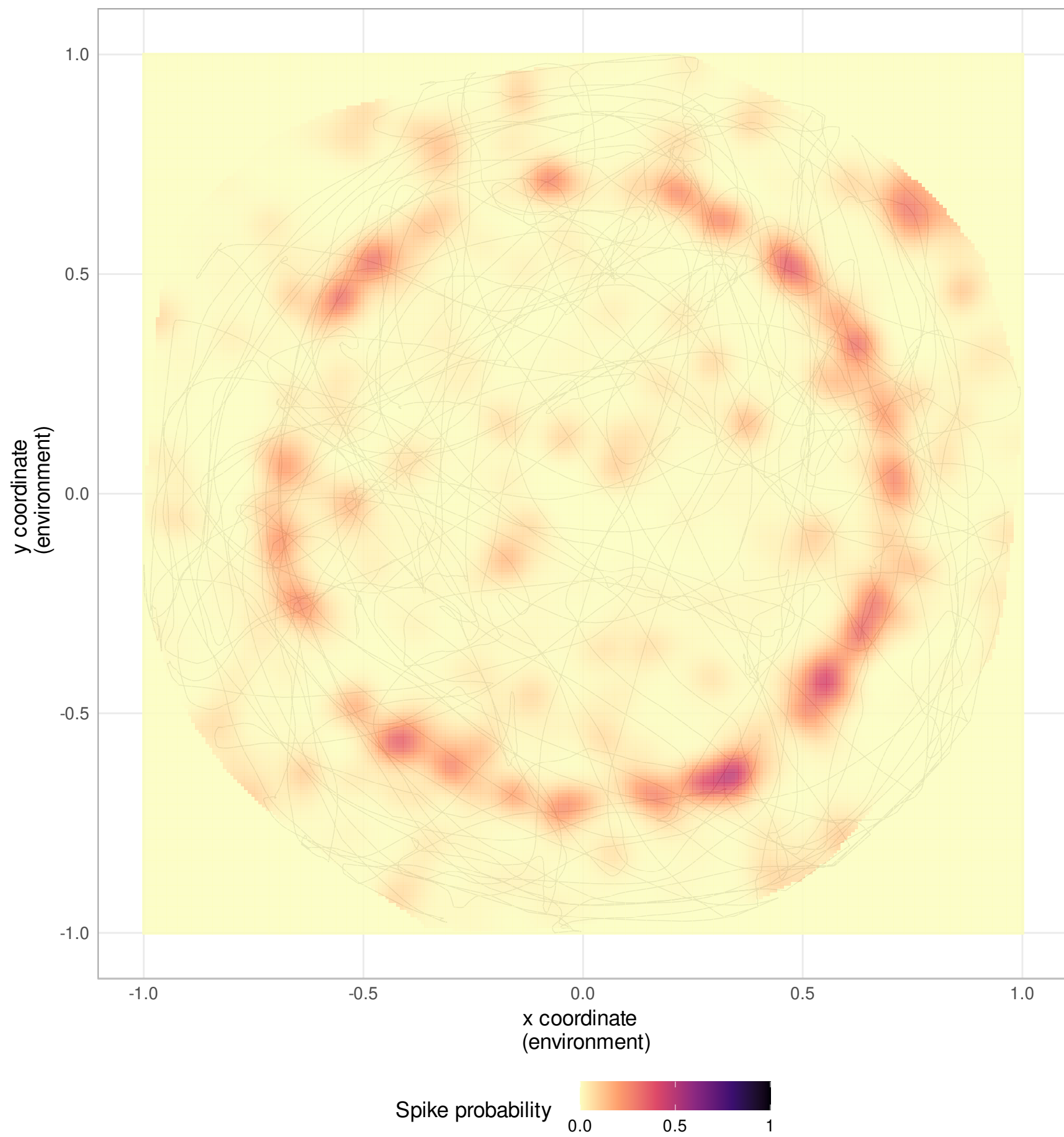
Neuron 288
