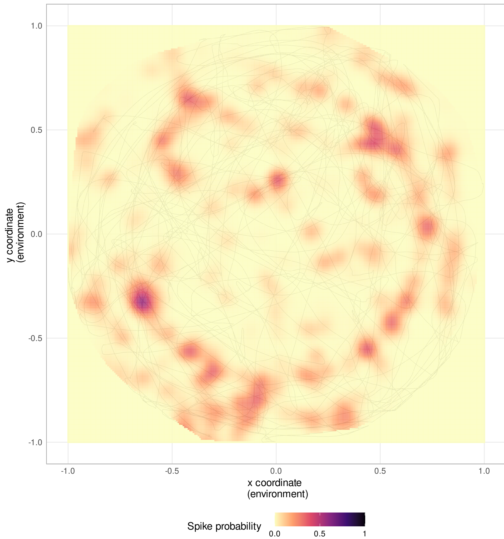
Neuron 291
