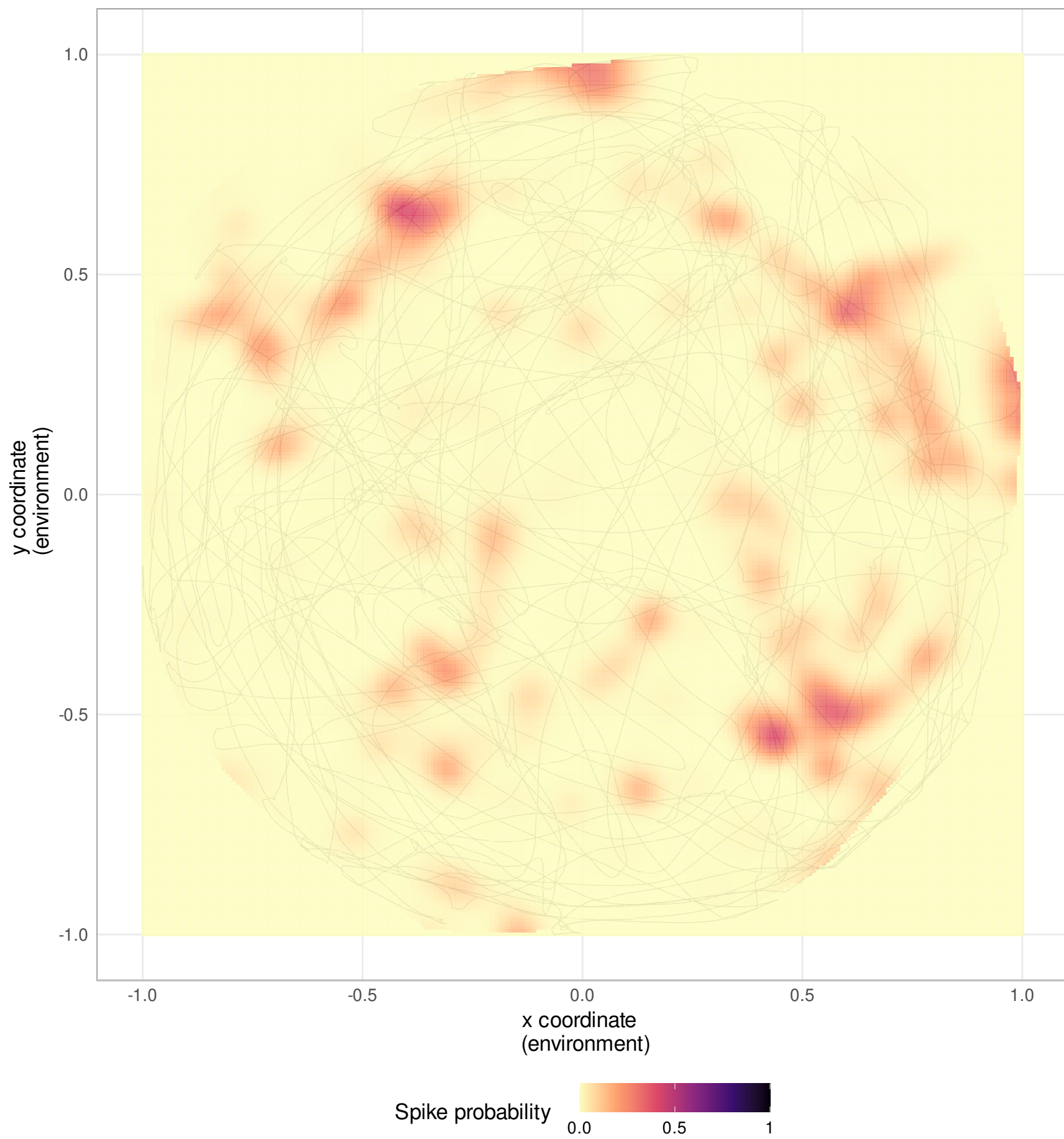
Neuron 292
