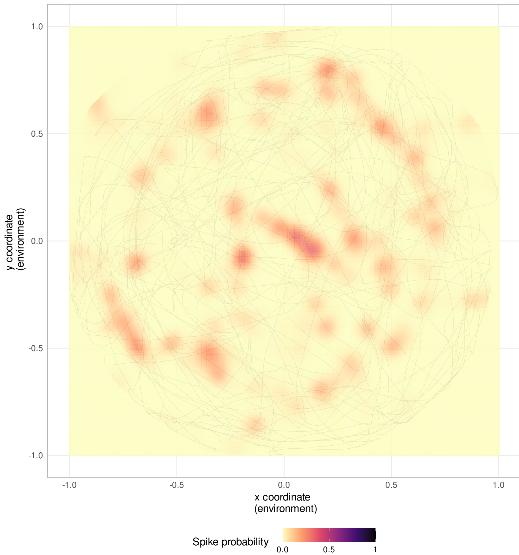
Neuron 298
