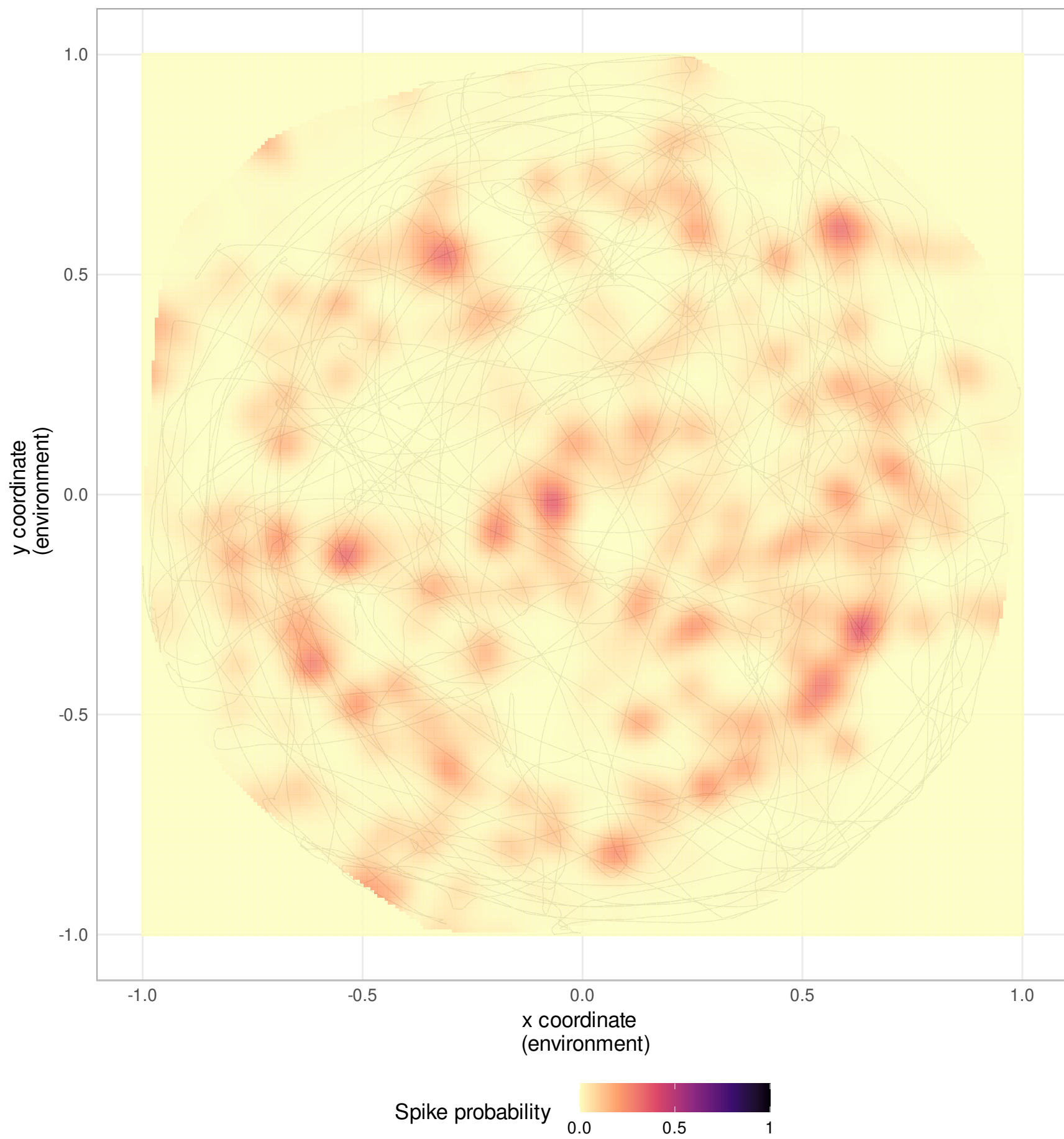
Neuron 299
