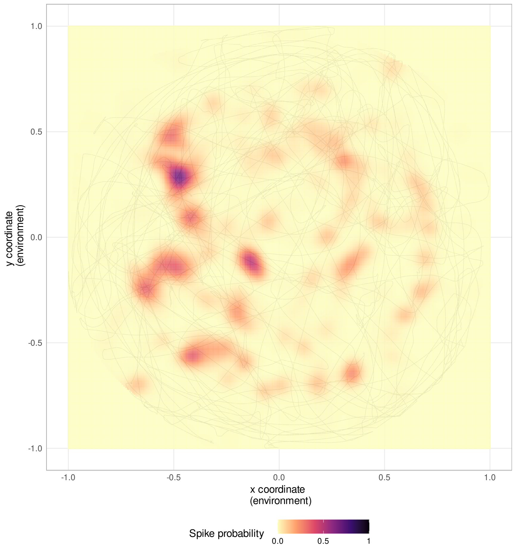
Neuron 302
