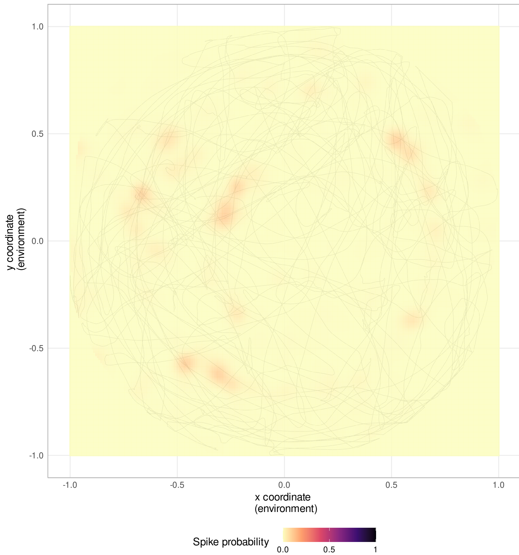
Neuron 305
