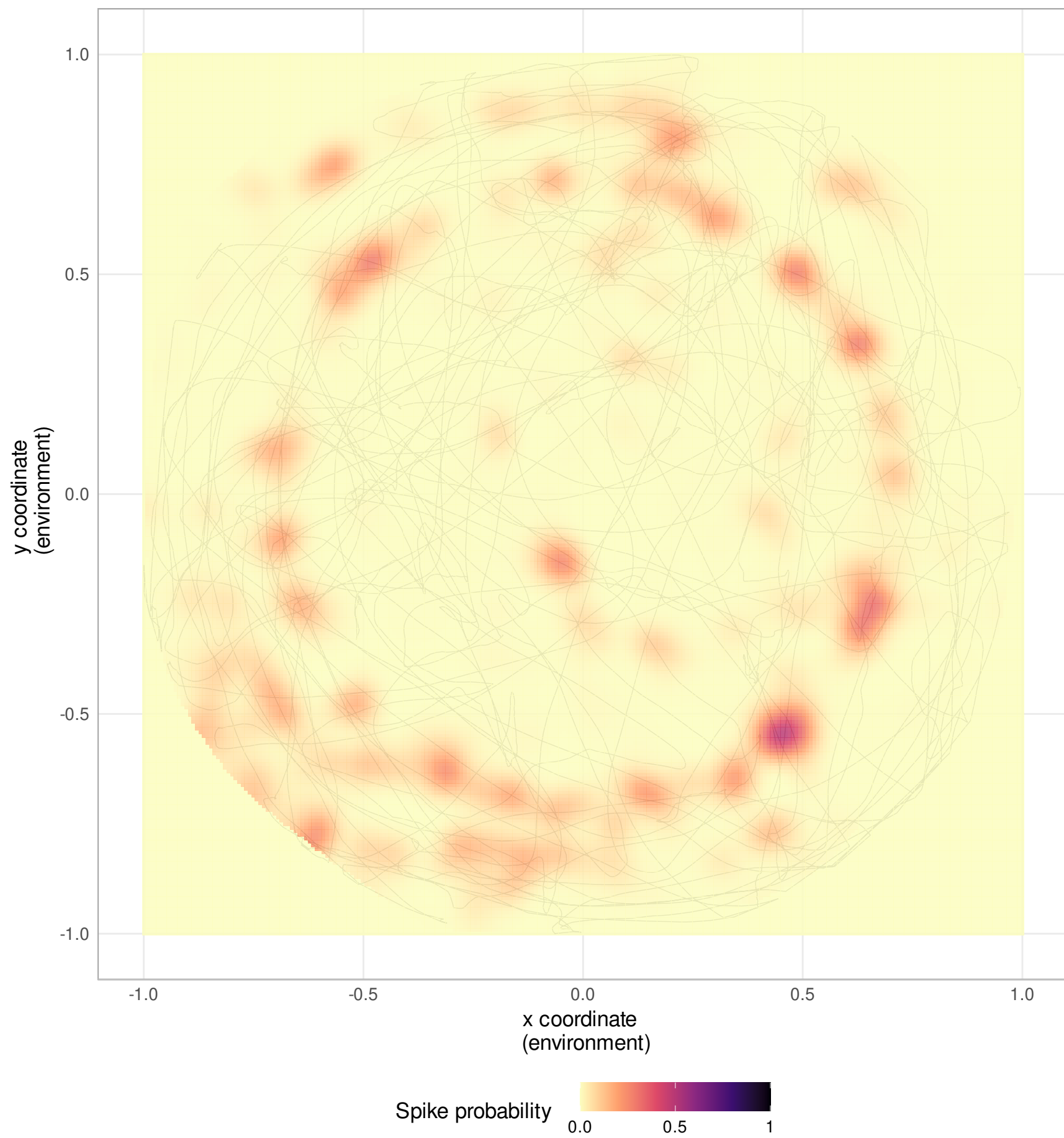
Neuron 307
