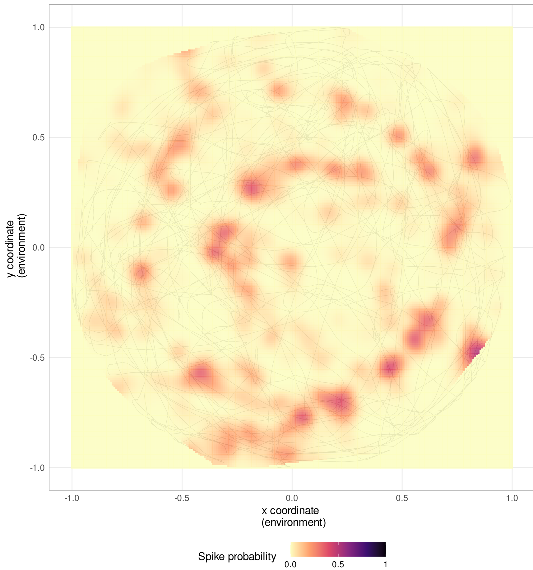
Neuron 309
