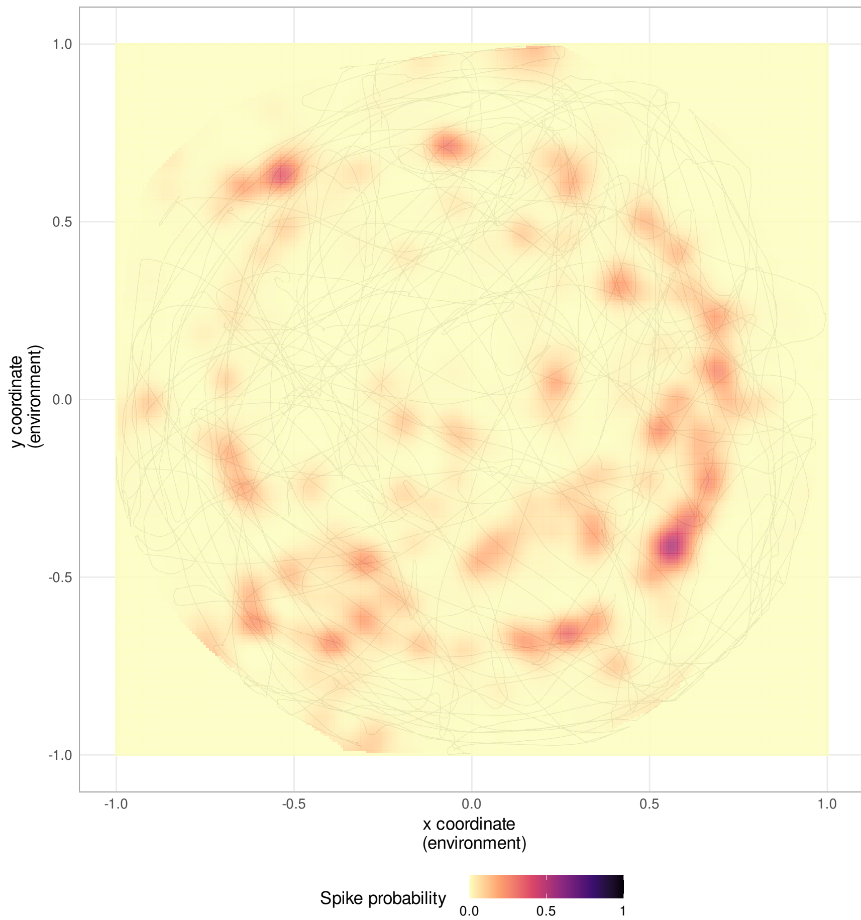
Neuron 313
