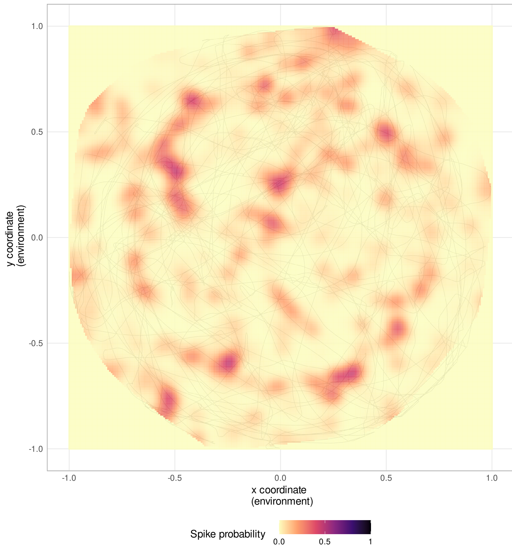
Neuron 321
