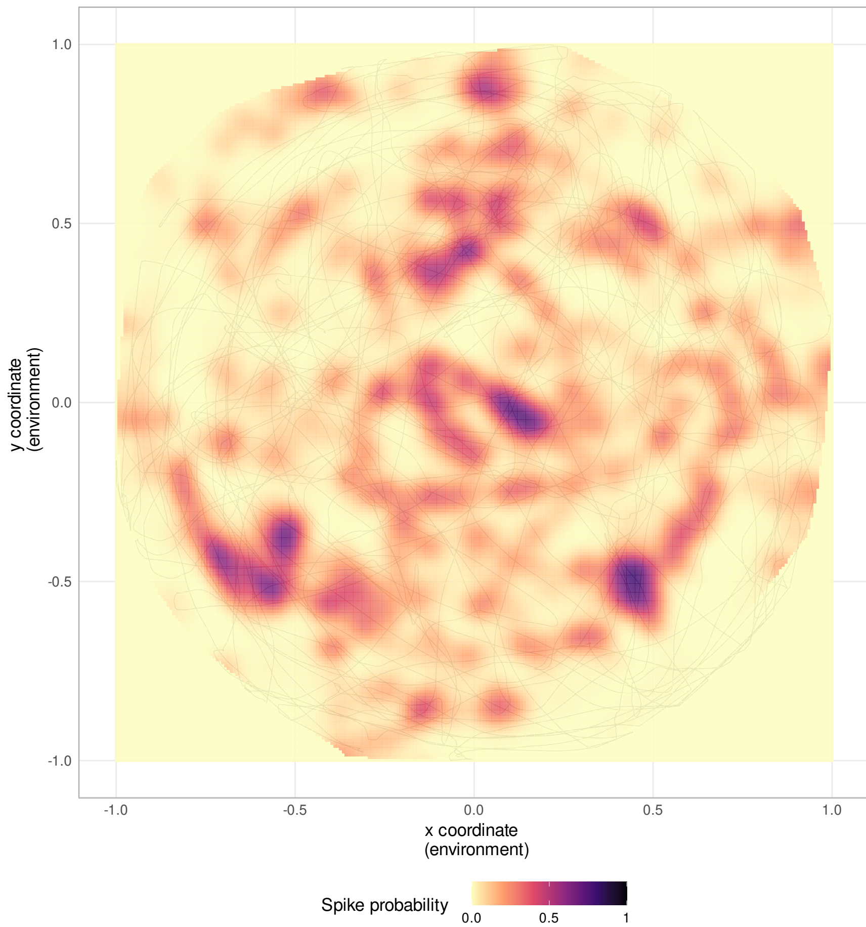
Neuron 33
