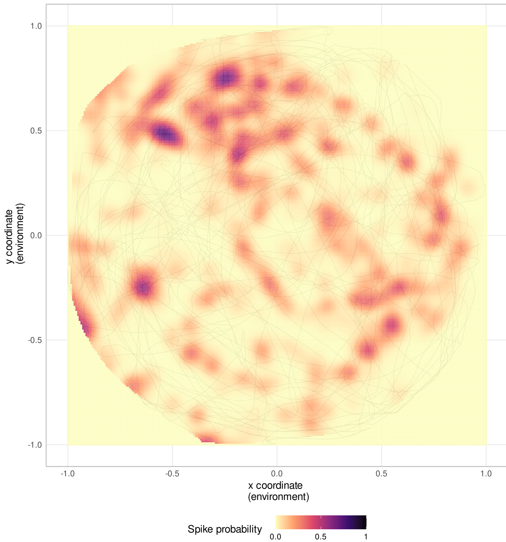
Neuron 54
