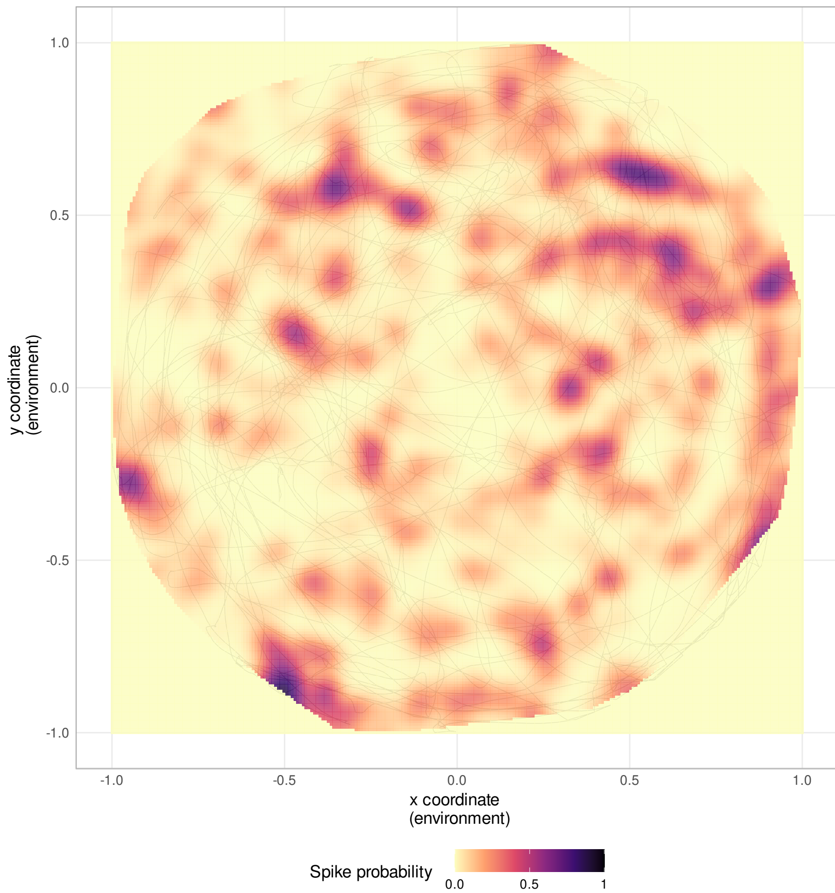
Neuron 6
