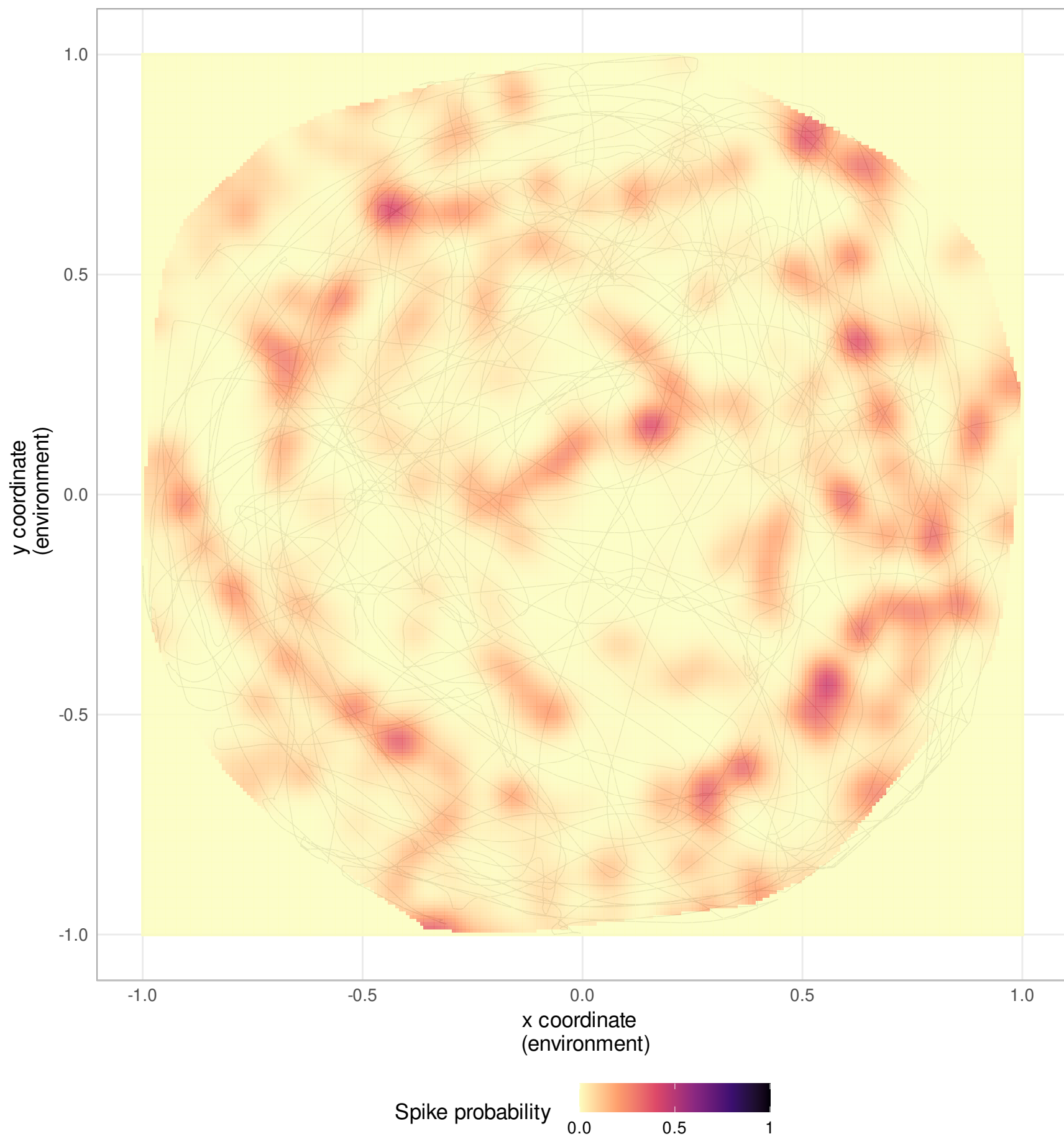
Neuron 82
