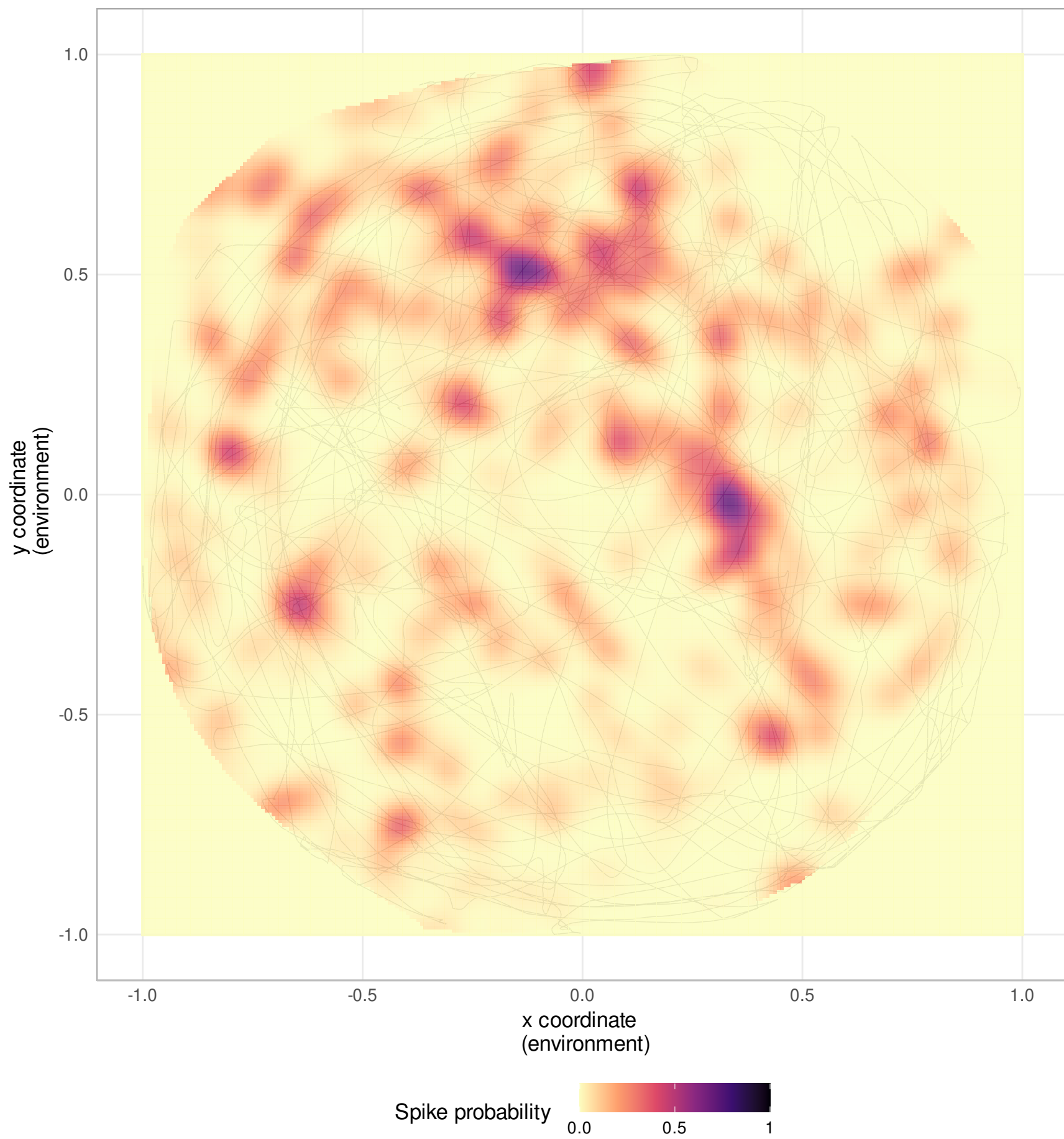
Neuron 96
