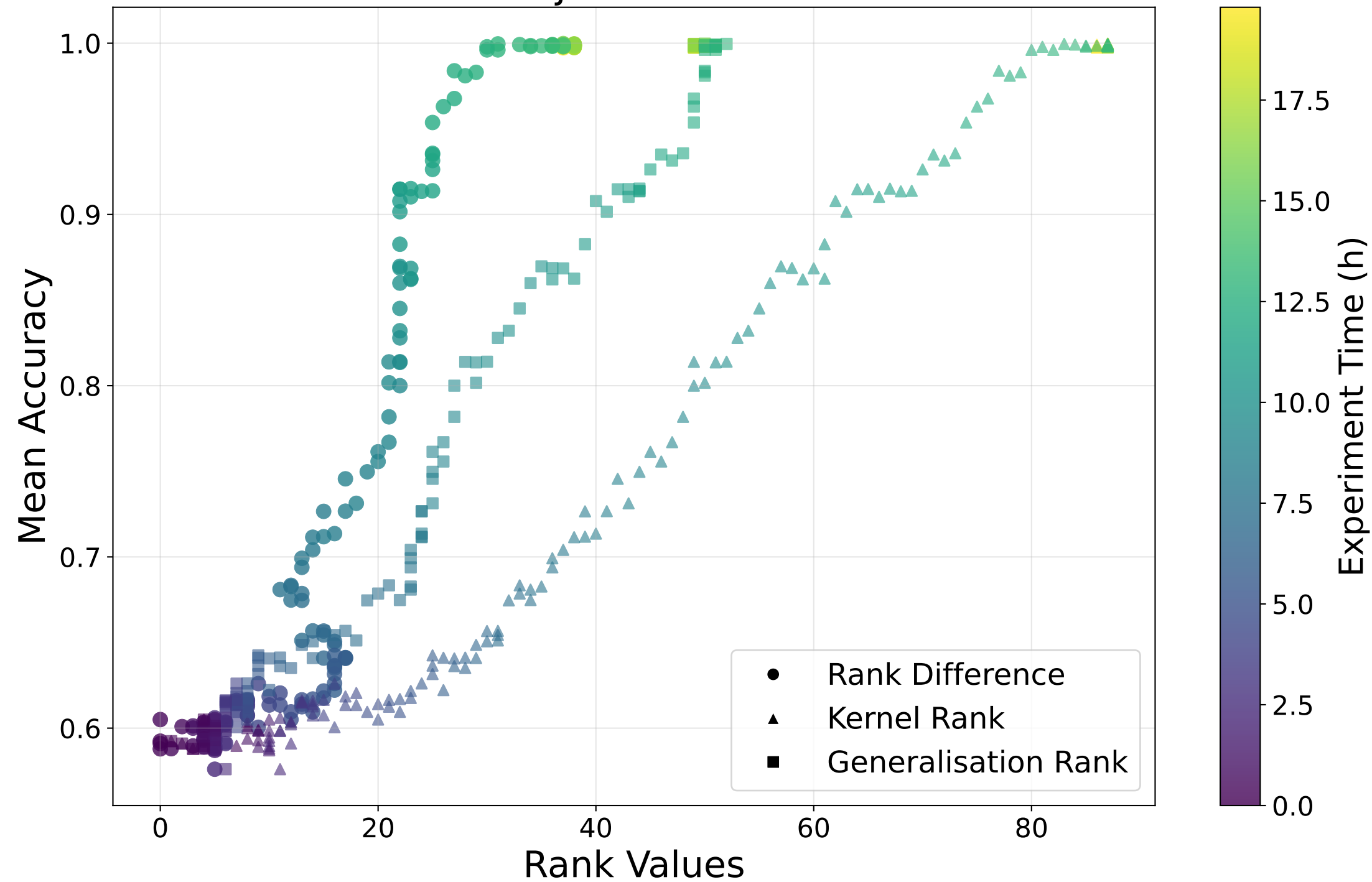
Rank Trajectories - E. coli
